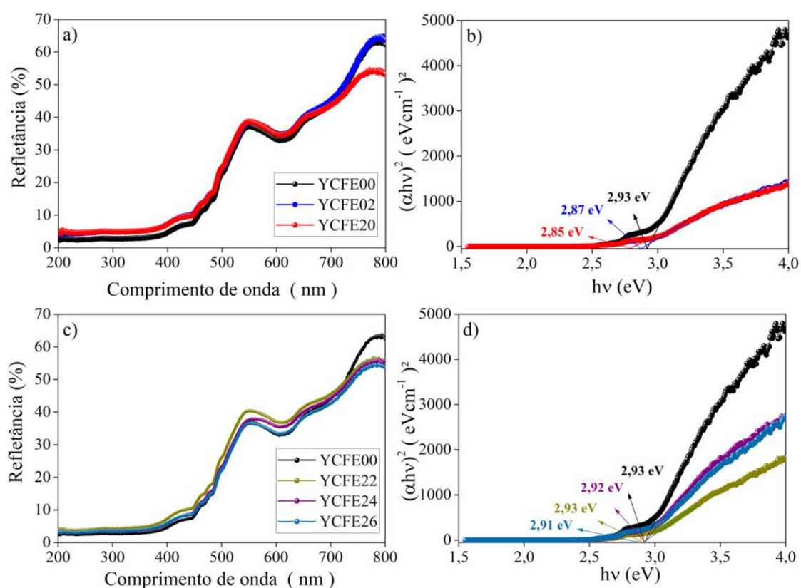
Figura 17 – Gráfico de Tauc para determinar o gap de energia no composto Y_{3-x}Ce_xFe_5-yEr_yO_{12} ( 0,00 \leq x \leq 0,02 ) e ( 0,00 \leq y \leq 0,06 ).
