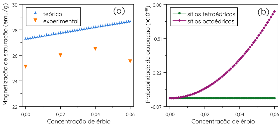
Figura 21 – Influência dos sítios de ocupação do dopante na magnetização de saturação do sistema Y_{2.98}Ce_{0.02}Fe_{5-y}Er_yO_{12} . a) Valores teóricos e experimentais de magnetização de saturação, M_s , em função do teor de cátions de Er^{3+} por fórmula unitária, y e b) Probabilidade de ocupação por sítio para os cátions de Er^{3+} , S_i^{Er^{3+}} , em função de teor de cátions de Er^{3+} por fórmula unitária, y .
