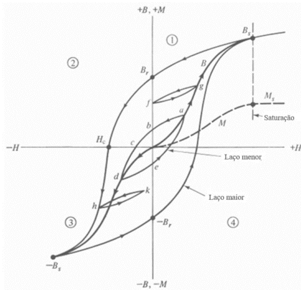
Figura 4 – Representação de curvas de magnetização
