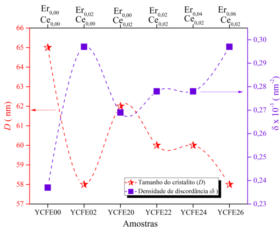
Figura 8 – Tamanho do cristalito e densidade de discordâncias do composto \text{Y}_{3-x}\text{Ce}_x\text{Fe}_{5-y}\text{Er}_y\text{O}_{12} , ( 0,00 \leq x \leq 0,02 ) e ( 0,00 \leq y \leq 0,06 ).
