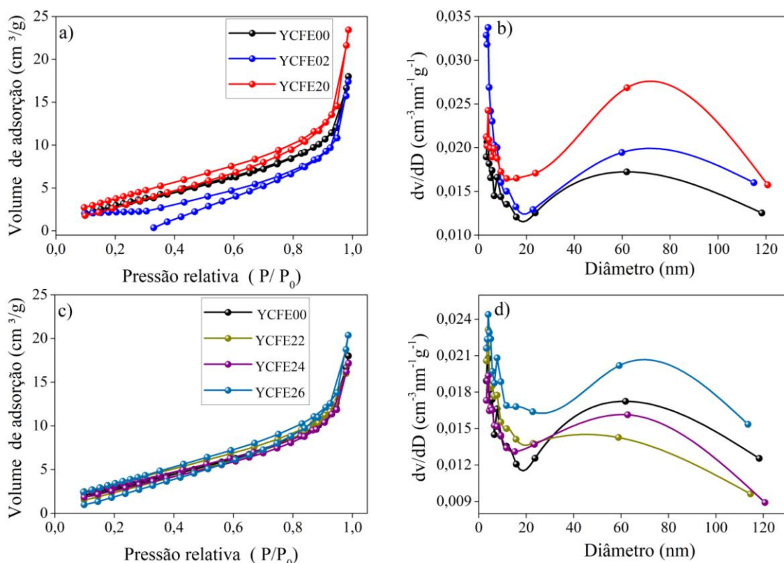
Figura 16 – Isotérmicas de adsorção-dessorção de nitrogênio do composto \text{Y}_{3-x}\text{Ce}_x\text{Fe}_{5-y}\text{Er}_y\text{O}_{12} ( 0,00 \leq x \leq 0,02 ) e ( 0,00 \leq y \leq 0,06 ).
