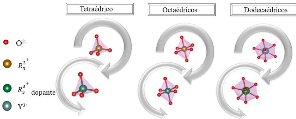
Figura 2 – Representação esquemática do processo de dopagem nos sítios cristalográficos no YIG ( Y_3Fe_5O_{12} ).
