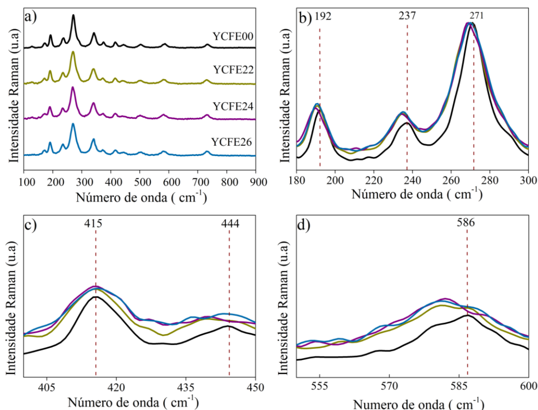
Figura 12 – Espectros Raman das amostras \text{Y}_{3-x}\text{Ce}_x\text{Fe}_{5-y}\text{Er}_y\text{O}_{12} , ( 0,00 \leq x \leq 0,02 ) e ( 0,00 \leq y \leq 0,06 ).
