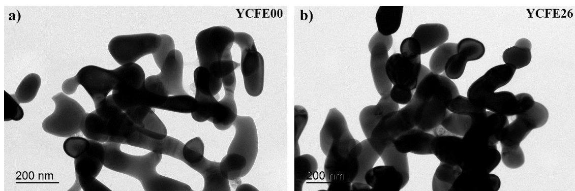
Figura 14 – Imagens MET para amostras YCFE00 e YCFE26
