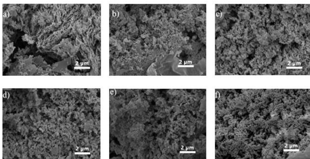
Figura 13 – Imagens de MEV das nanopartículas do composto Y_{3-x}Ce_xFe_{5-y}Er_yO_{12} , (0,00 \leq x \leq 0,02) e (0,00 \leq y \leq 0,06)
