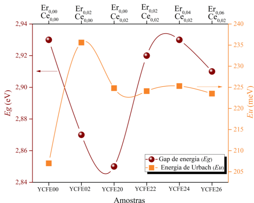
Figura 19 – Gap de energia ótico e energia Urbach do composto Y_{3-x}Ce_xFe_{5-y}Er_yO_{12} ( 0,00 \leq x \leq 0,02 ) e ( 0,00 \leq y \leq 0,06 ).
