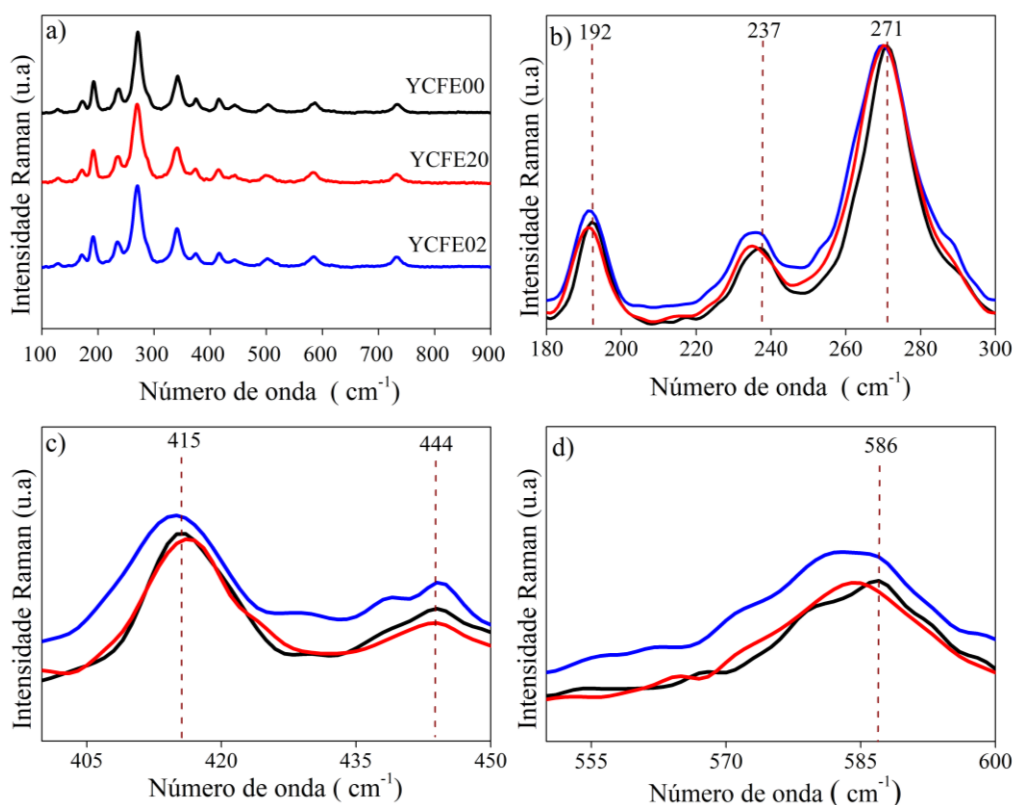
Figura 11 – Espectros Raman das amostras \text{Y}_{3-x}\text{Ce}_x\text{Fe}_{5-y}\text{Er}_y\text{O}_{12} , ( 0,00 \leq x \leq 0,02 ) e ( 0,00 \leq y \leq 0,02 ).
