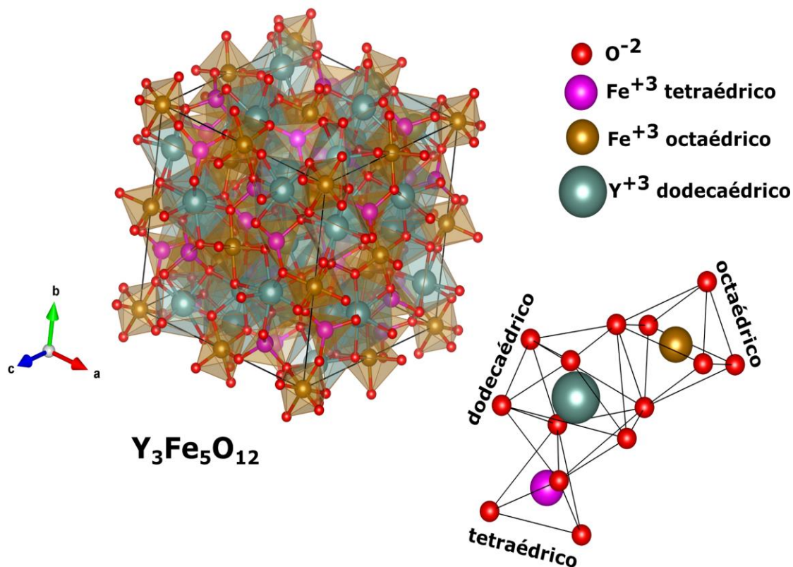
Figura 1 – Representação da granada de ferro ítrio com seus sítios cristalográficos. 23 jun. 2021. Software Vesta.
