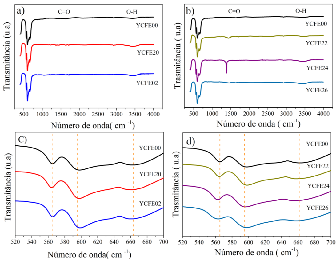
Figura 10 – Espectros FTIR do composto Y_{3-x}Ce_xFe_{5-y}Er_yO_{12} , ( 0,00 \leq x \leq 0,02 ) e ( 0,00 \leq y \leq 0,06 ).
