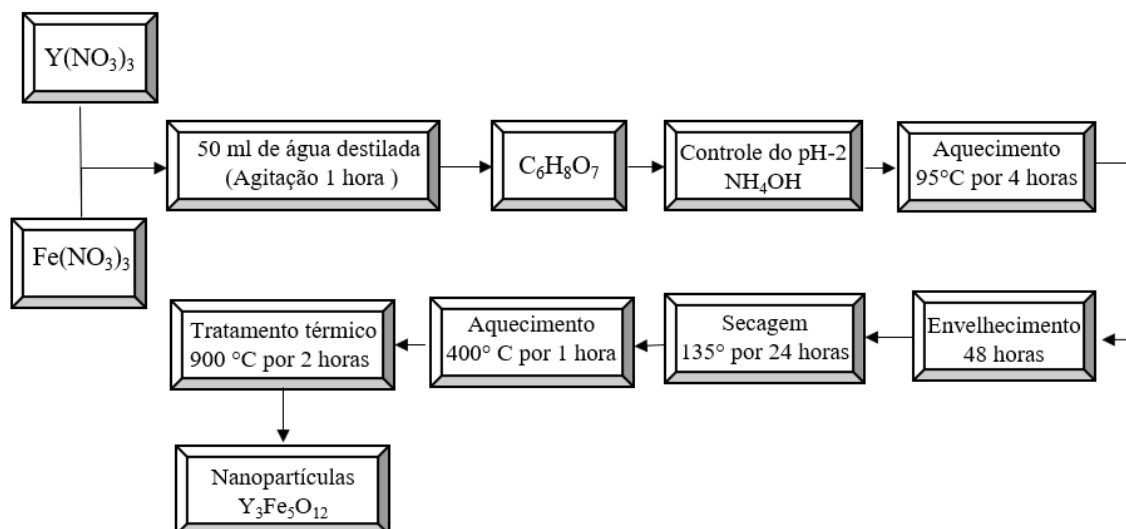
Figura 6 – Representação esquemática do processo de síntese do composto Y_{3-x}Ce_xFe_{5-y}Er_yO_{12} , ( 0,00 \leq x \leq 0,02 ) e ( 0,00 \leq y \leq 0,06 ).
