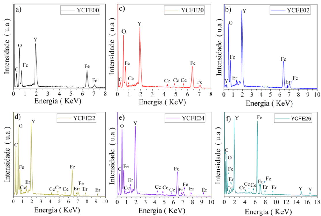
Figura 15 – Espectros de EDS do composto \text{Y}_{3-x}\text{Ce}_x\text{Fe}_{5-y}\text{Er}_y\text{O}_{12} , ( 0,00 \leq x \leq 0,02 ) e ( 0,00 \leq y \leq 0,06 ).
