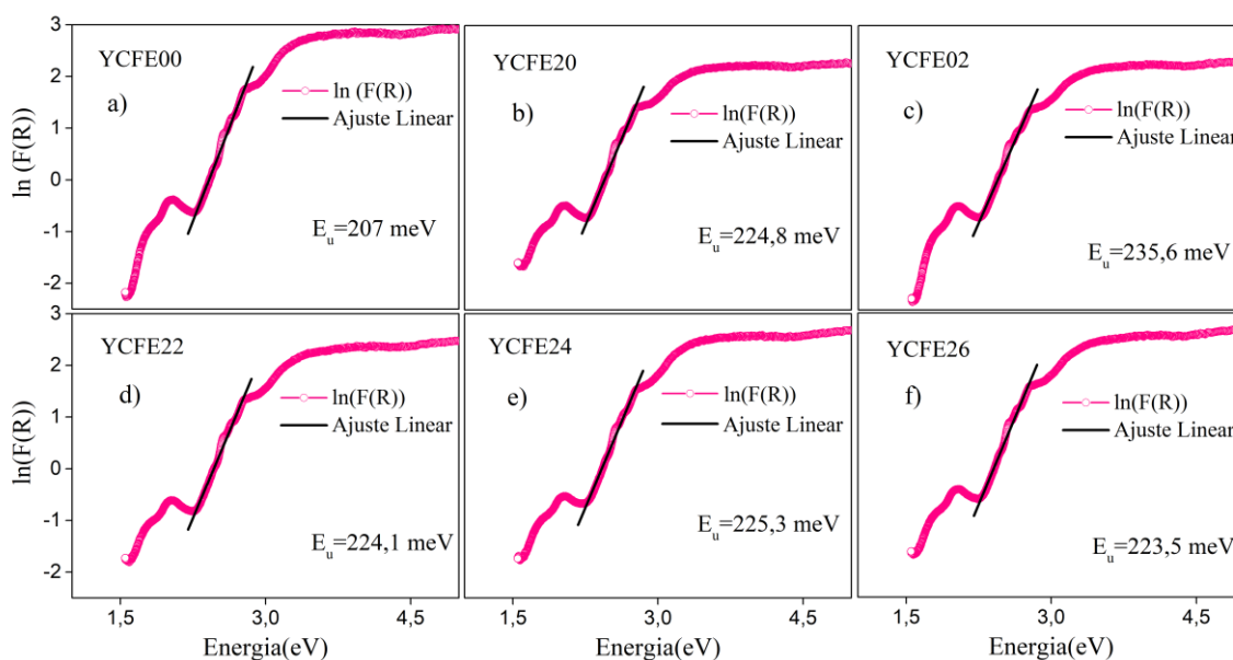
Figura 18 – \ln(F(R)) vs Energia ( h\nu ) do composto Y_{3-x}Ce_xFe_{5-y}Er_yO_{12} ( 0,00 \leq x \leq 0,02 ) e ( 0,00 \leq y \leq 0,06 ).
