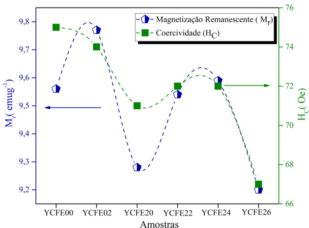
Figura 23 – Magnetização de remanescente e coercividade de nanopartículas do composto \text{Y}_{3-x}\text{Ce}_x\text{Fe}_{5-y}\text{Er}_y\text{O}_{12} ( 0,00 \leq x \leq 0,02 ) e ( 0,00 \leq y \leq 0,06 ).
