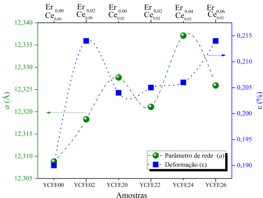
Figura 9 – Parâmetro de rede e deformação da rede do composto \text{Y}_{3-x}\text{Ce}_x\text{Fe}_{5-y}\text{Er}_y\text{O}_{12} , ( 0,00 \leq x \leq 0,02 ) e ( 0,00 \leq y \leq 0,06 ).
