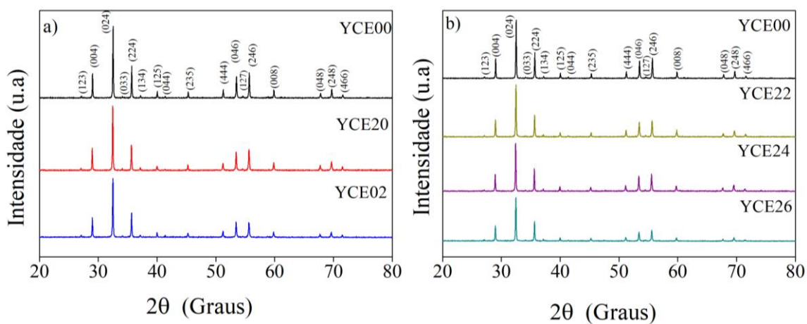
Figura 7 – Padrões de difração de raios-X do composto \text{Y}_{3-x}\text{Ce}_x\text{Fe}_{5-y}\text{Er}_y\text{O}_{12} , ( 0,00 \leq x \leq 0,02 ) e ( 0,00 \leq y \leq 0,06 ). a) YIG puro e dopado, b) YIG puro e co-dopado.
