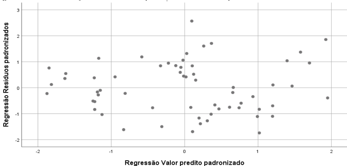
Figura 3 - Gráfico da relação entre os resíduos padronizados e os valores previstos de DISA
