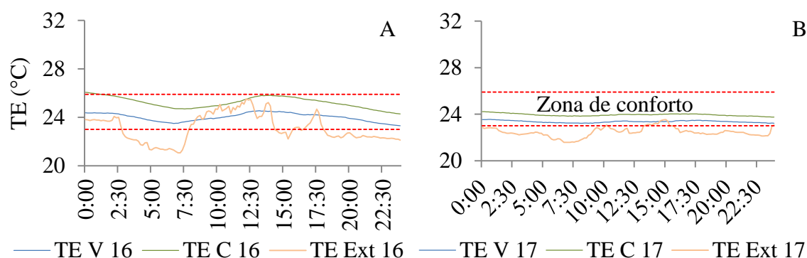
Figura 14: Variação diária do índice de TE no interior das salas e no ambiente externo para o dia crítico de menor temperatura, antes e após implantação do telhado verde, 09/08/2016 (A) e 19/07/2017 (B), respectivamente.
