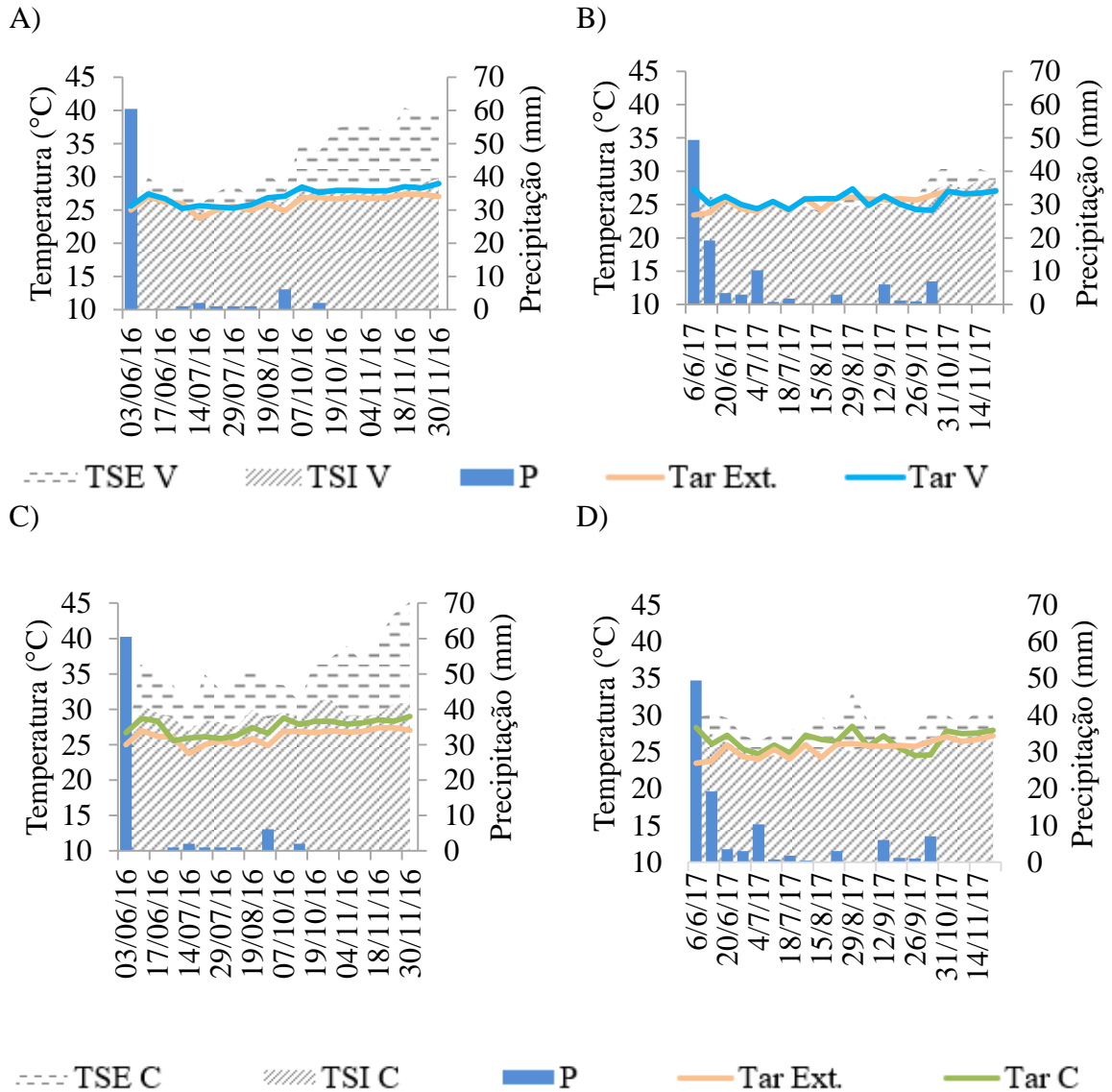
Figura 18: Precipitação acumulada (P), média diária da temperatura superficial externa e interna da cobertura da sala de vidro (TSE V e TSI V), temperatura do ar do ambiente externo (Tar Ext.) e temperatura do ar no interior da sala de vidro (Tar V), para o período (A) sem telhado verde; (B) com telhado verde. Precipitação acumulada (P), média diária da temperatura superficial externa e interna da cobertura da sala de compensado (TSE C e TSI C), temperatura do ar do ambiente externo (Tar Ext.) e temperatura do ar interna da sala de compensado (Tar C), para o período (C) sem telhado verde; (D) com telhado verde.
