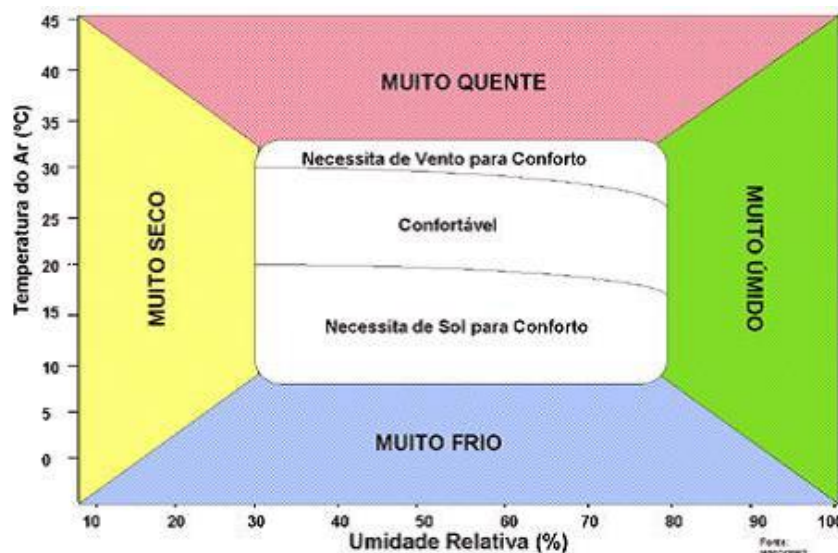
Figura 5: Diagrama do conforto humano. Fonte: INMET (2017).
