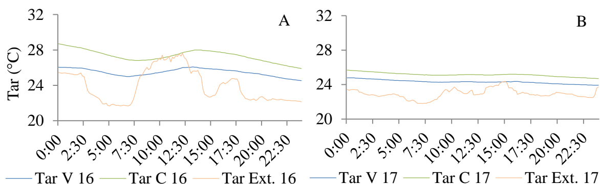
Figura 13: Temperatura do ar no ambiente externo e nas salas, para o dia crítico de menor temperatura, antes e após implantação do telhado verde, 09/08/2016 (A) e 19/07/2017 (B), respectivamente.
