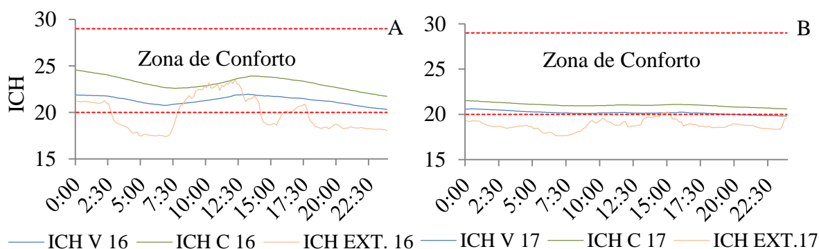
Figura 15: Variação diária do ICH no interior das salas e no ambiente externo para o dia crítico de menor temperatura, antes e após implantação do telhado verde, 09/08/2016 (A) e 19/07/2017 (B), respectivamente.
