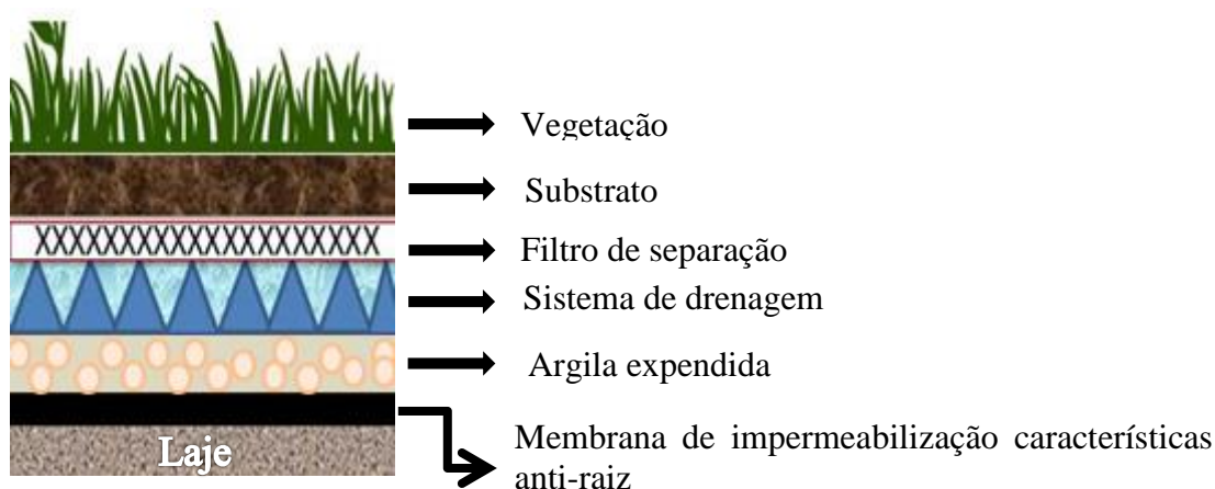
Figura 4: Representação esquemática da estrutura geral de um telhado verde. Fonte: Autor, 2017.
