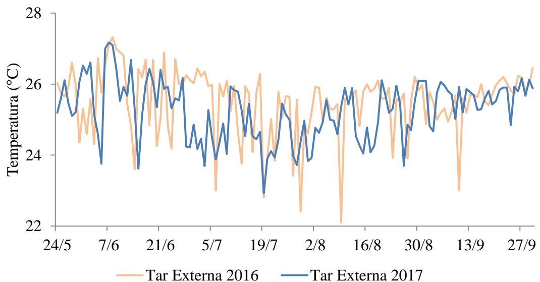
Figura 9: Média diária da temperatura do ar do ambiente externo no período de 24/05 a 30/09 de 2016 e 2017. Tar Externa 2016 – Temperatura do ar externa em 2016; Tar Externa 2017 – Temperatura do ar externa em 2017.
