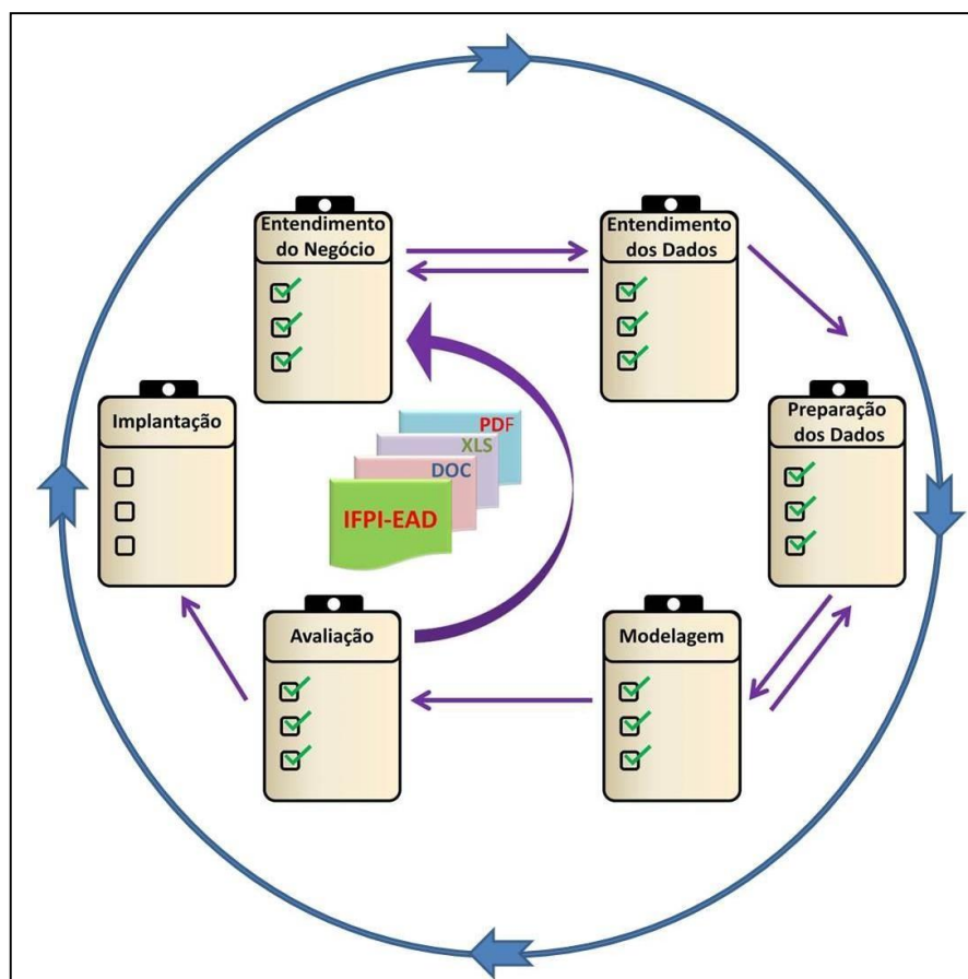
Figura 5 - Metodologia CRISP-DM aplicada a EAD do IFPI
