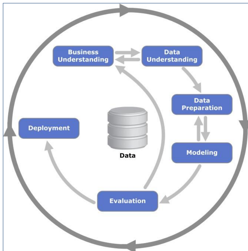
Figura 3 – Metodologia CRISP-DM
