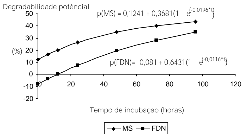
Figura 1. Cinética da degradação da matéria seca (MS) e da fibra em detergente neutro (FDN) do feno de capim-de-raiz no rúmen de caprinos.
