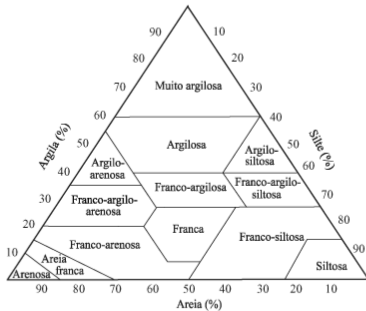
Figura 8. Triângulo de classificação textural de solos (LEMOS & SANTOS, 1996).
