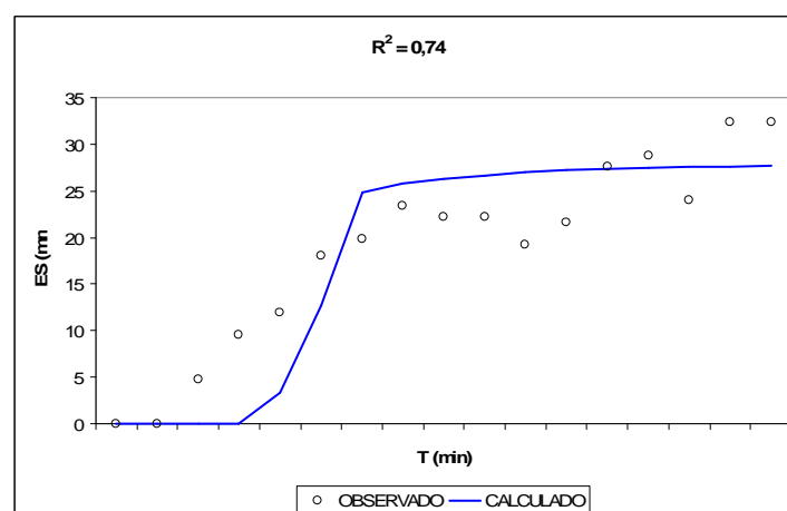
FIGURA 17 - Calibração da Vazão para os eventos NB2 11, NB2 12 e NB2 13 respectivamente da BRM em parcela experimental.
