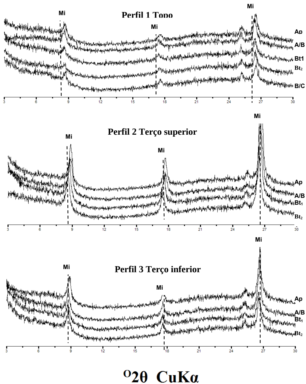
Figura 4. Difratomogramas das argilas saturadas com potássio (550°C). Mi = Mica (Ilita).
