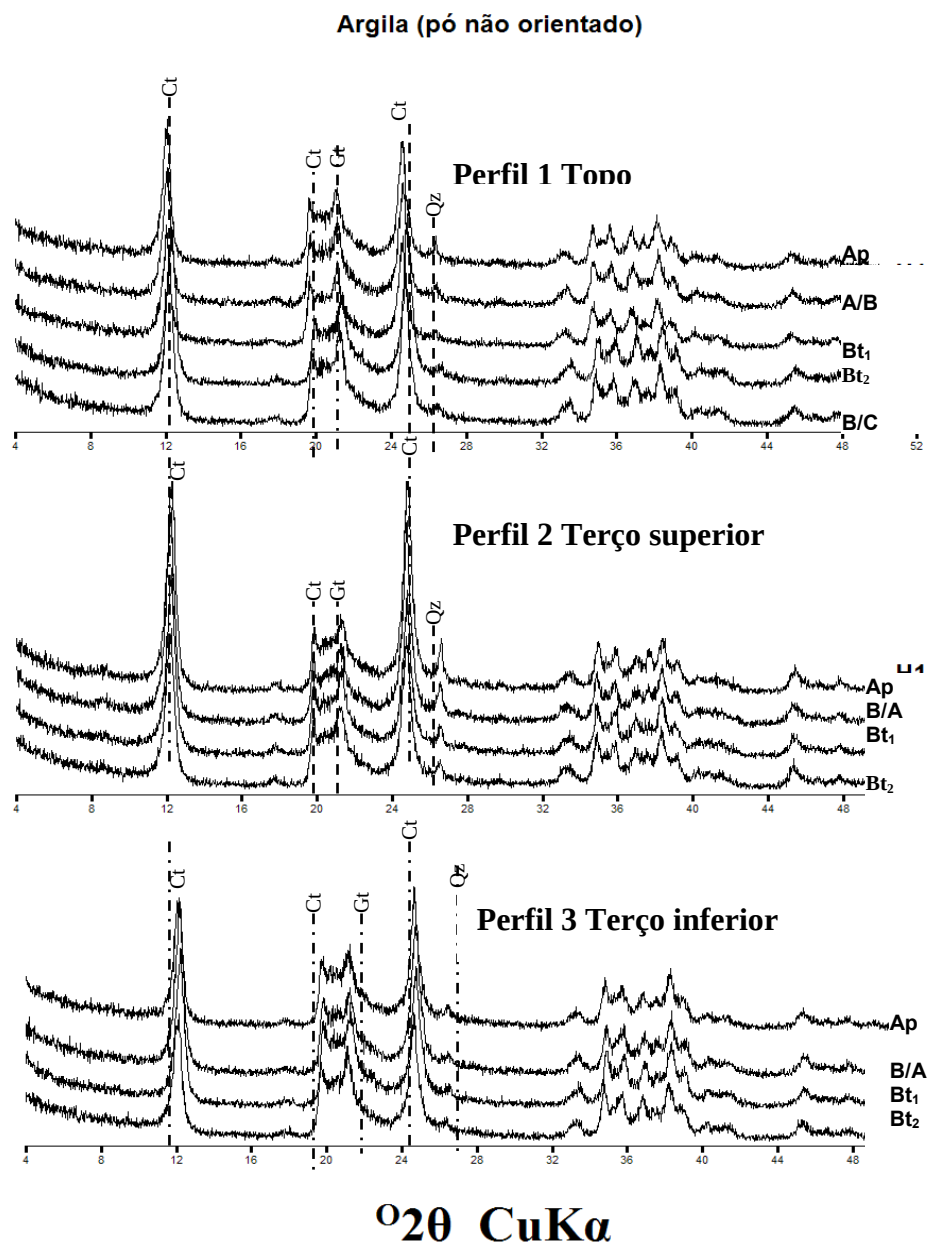
Figura 2. Difratomogramas das argilas sem tratamento químico. Ct = caulinita, Gt = goethita, Qz = quartzo.
