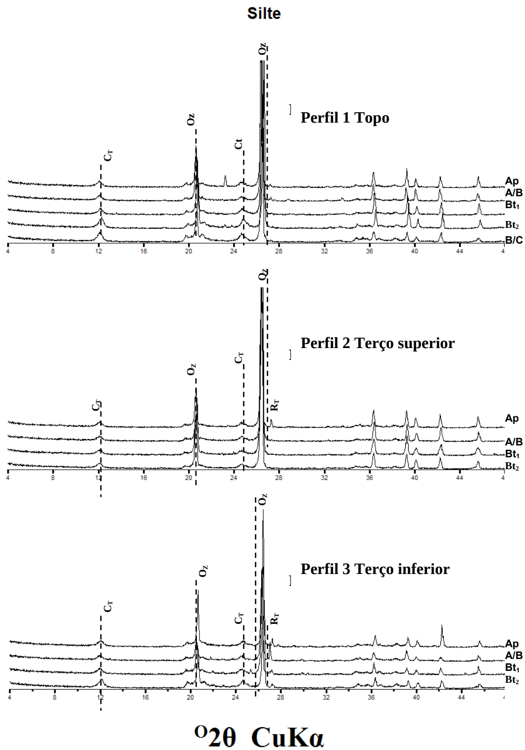
Figura 5. Difractogramas do silte sem tratamento químico. Ct = caulinita, Qz = quartzo, Rt = rutile.
