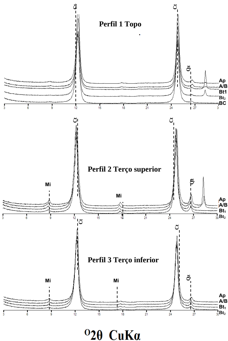
Figura 3. Difractogramas das argilas saturadas com potássio (25°C). Ct = caulinita, Qz = quartzo.
