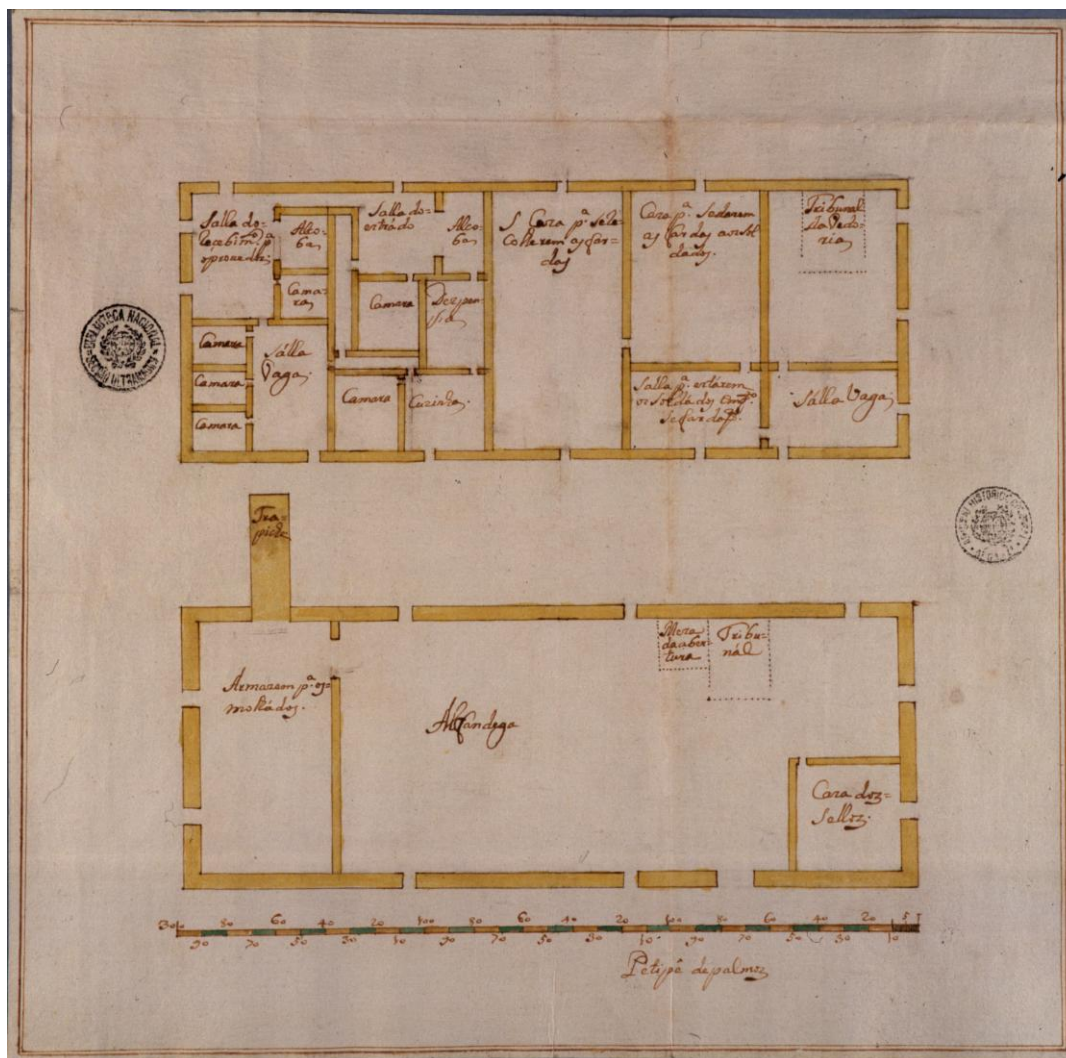
Figura (10): Planta da nova alfândega de Pernambuco, no Forte do Matos. [1732]. 822
