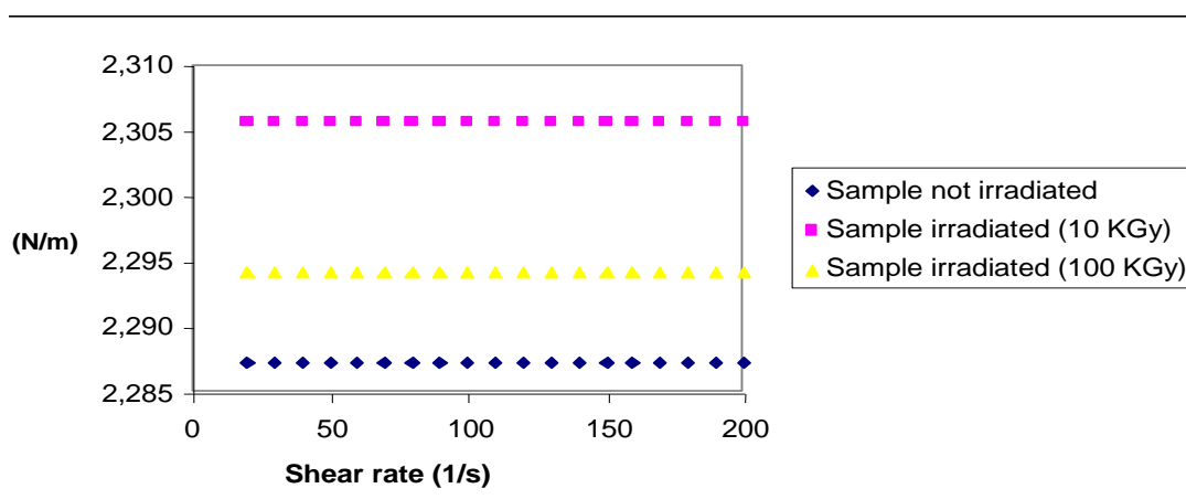
Figura 1 – Análise reológica do gel mediante diferentes condições. Podendo ser observada a viscosidade aparente, que é aquela medida em um único ponto através de cisalhamento constante. Observando-se uma redução da viscosidade com o aumento da dose de irradiação.
