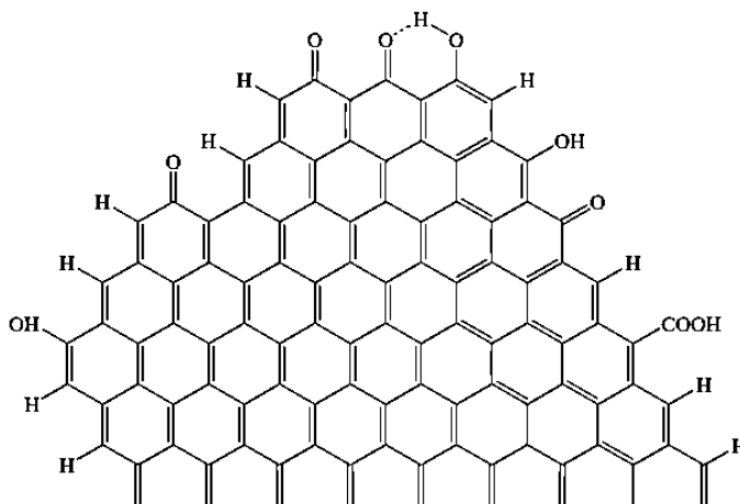
Figura 14. Estrutura química do negro-de-fumo.
