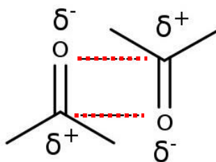
Figura 10. Interação dipolo-dipolo entre duas moléculas de propanona.
