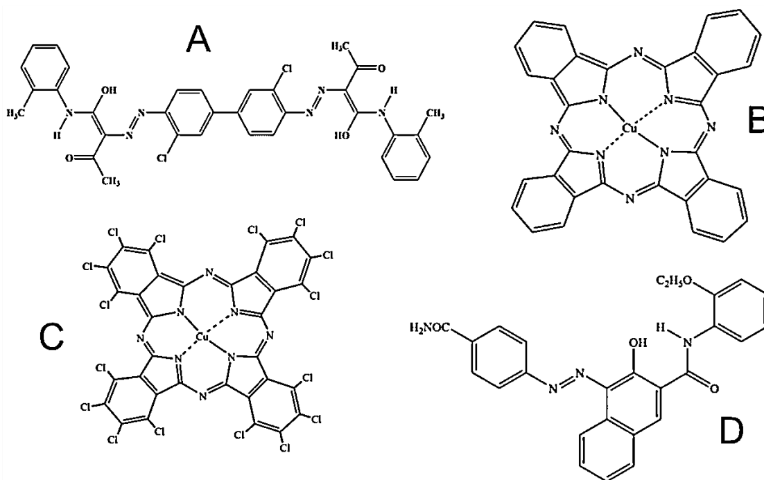
Figura 15. Estrutura química dos pigmentos do tipo orgânico.
