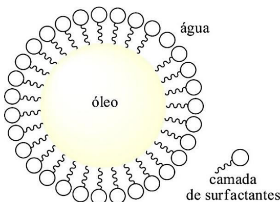
Figura 12. Representação de uma micela globular com camadas surfactantes com parte lipofílica interna e hidrofílica externa.
