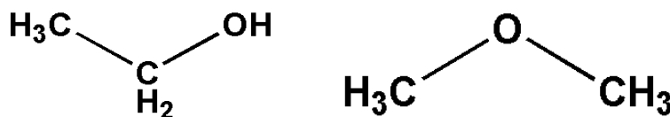
Figura 11. Estruturas moleculares do álcool etílico e éter dimetílico.
