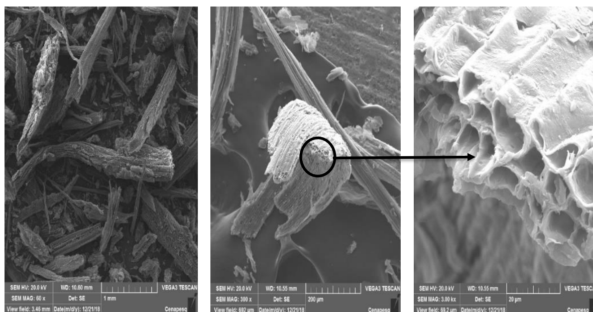
Figura 5: Imagens da Microscopia de Eletrônica de Varredura para o BC500 com ampliações de 60x, 300x e 3000x, respectivamente.
