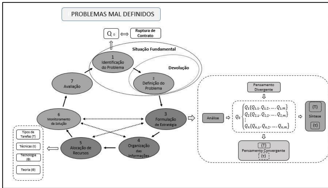
Figura 10 - Algumas Relações entre o PEP e o CSP
