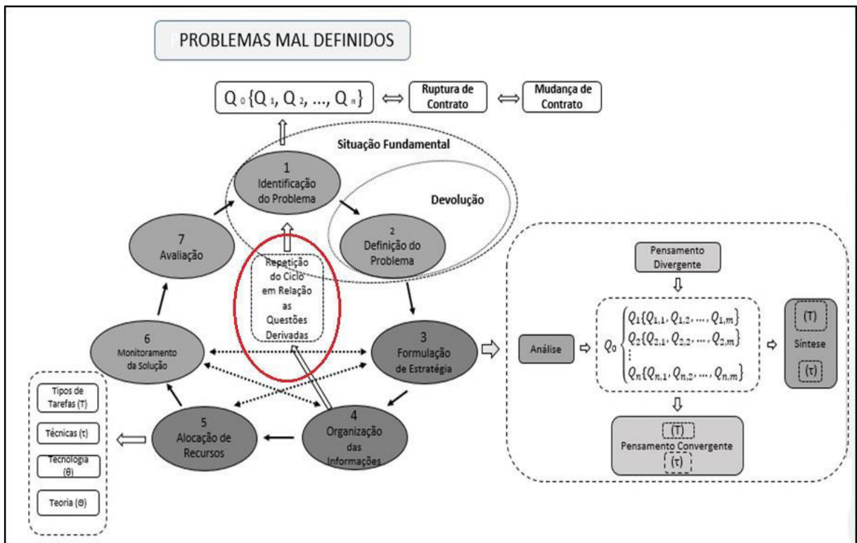
Figura 122 - Ciclo de Solução de Problemas Confirmando a Repetição dos Passos
