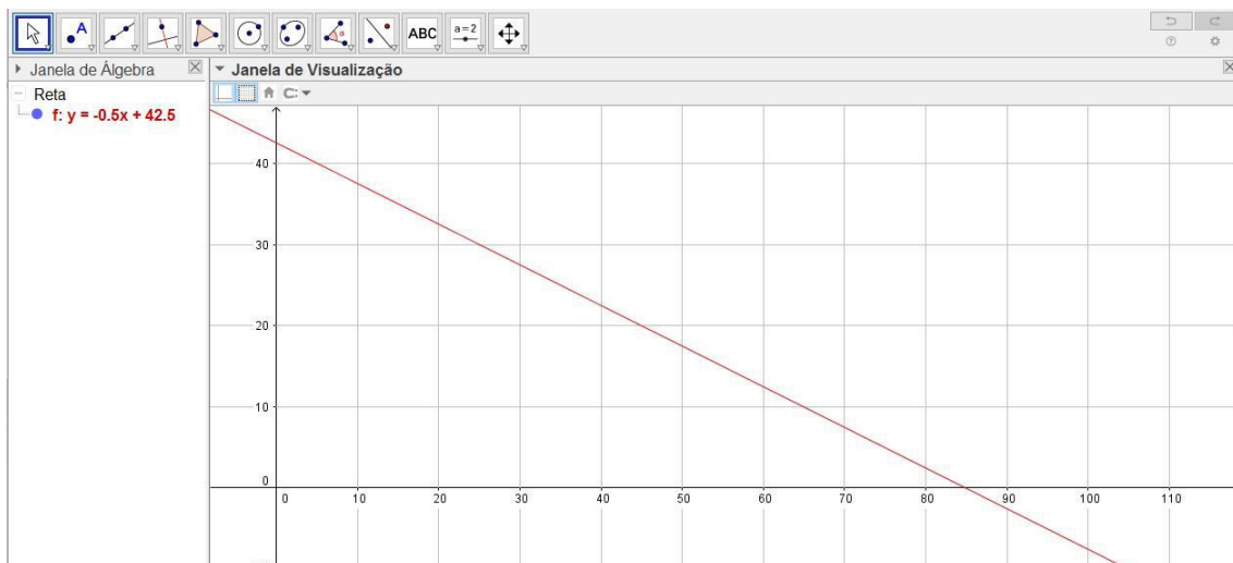
Figura 36 - Função Tempo de Contribuição (TC)
