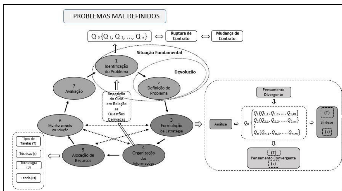
Figura 11 - Repetição do CSP na aplicação do PEP
