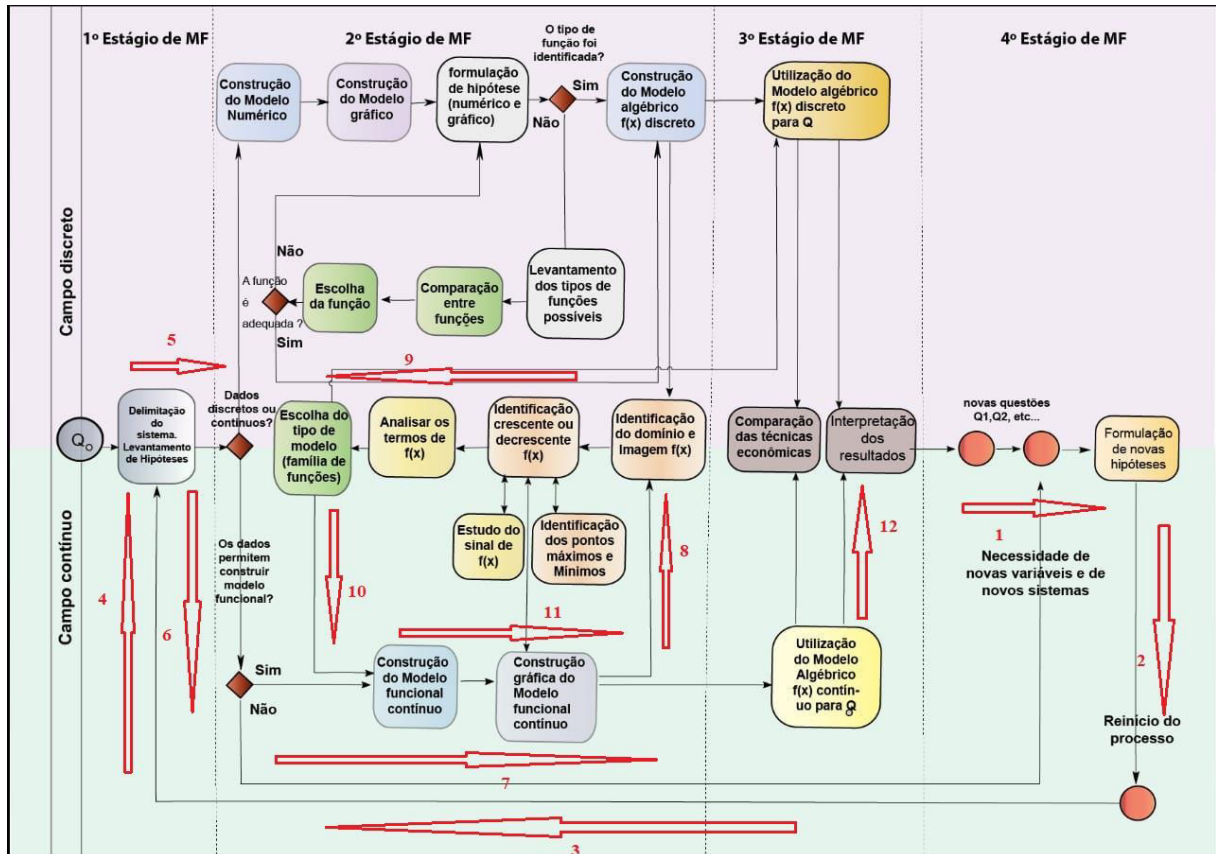
Figura 121 - Percurso dos Grupos durante o Sexto Encontro Presencial do Segundo Estudo Empírico
