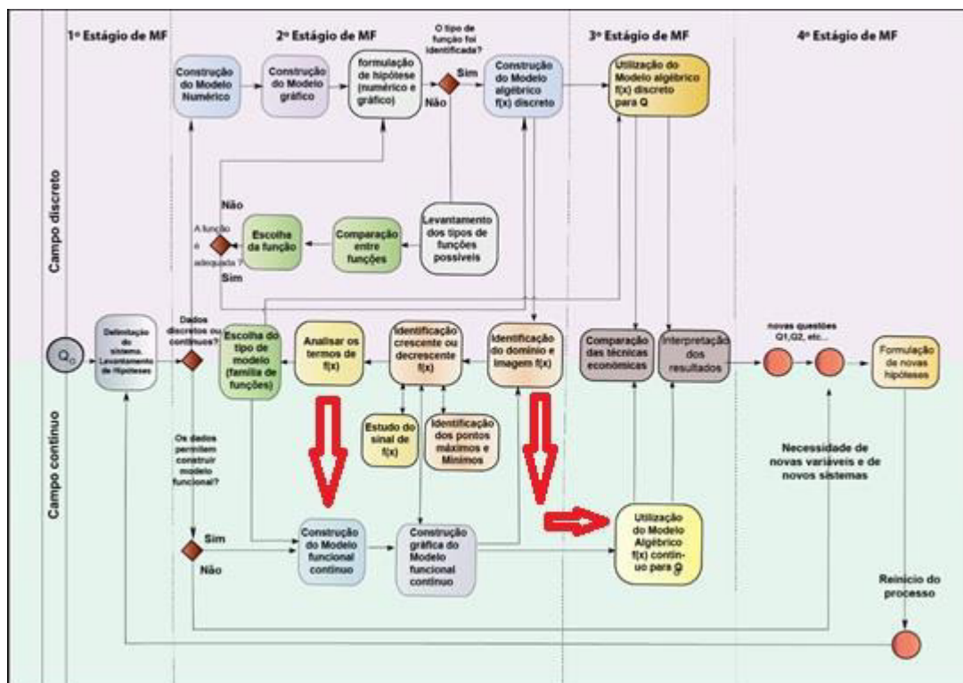
Figura 123 - Mudanças do Diagrama para o Ensino de Função na Licenciatura em Matemática
