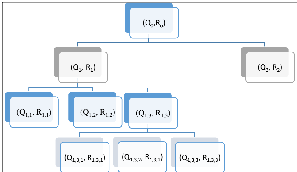
Figura 40 - Desenvolvimento de Q_1
