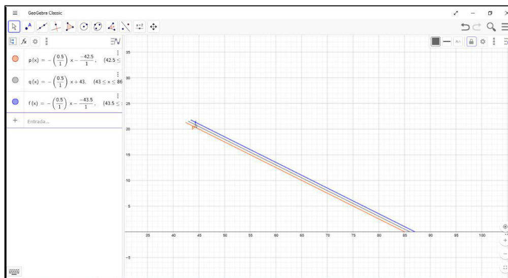
Figura 120 - Família da Função TC Construída por um dos Grupos
