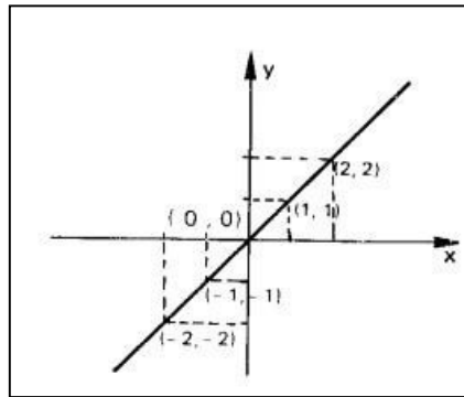
Figura 19 - Função Identidade
