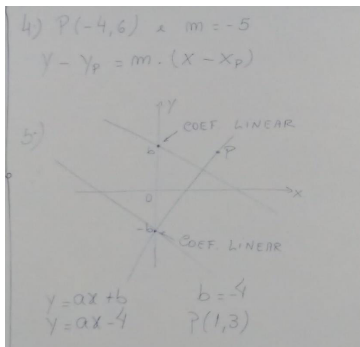
Figura 100 - Explicação do Item 04 pelo Professor
