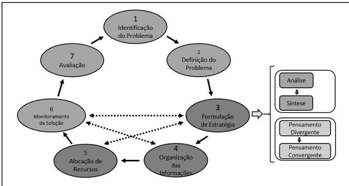
Figura 6 - Ciclo de Solução de Problemas
