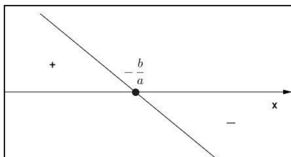
Figura 29 - Representação gráfica quando a < 0
