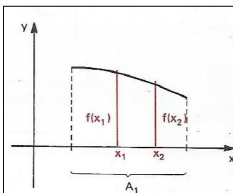
Figura 26 - Função Decrescente
