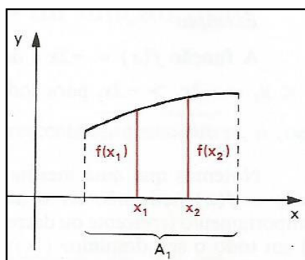
Figura 25 - Função Crescente
