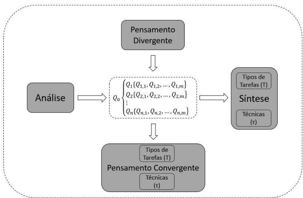
Figura 9 - Representação do Processo de Resolução do PEP pelo terceiro passo do Ciclo de Solução de Problemas
