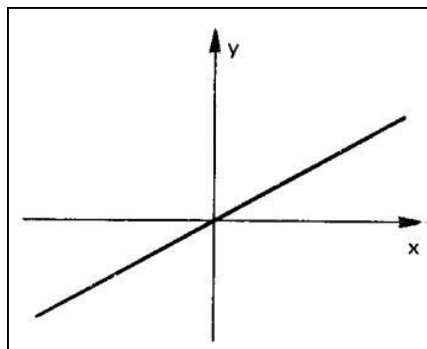
Figura 20 - Função Linear
