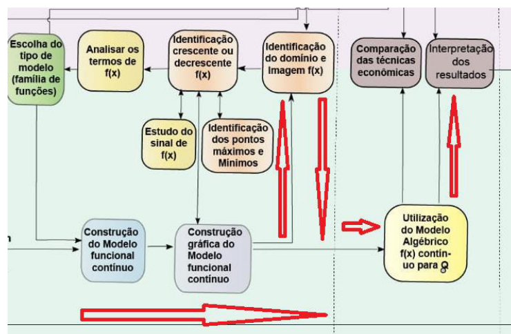
Figura 116 - Percurso do nosso MER em relação ao Encontro Presencial
