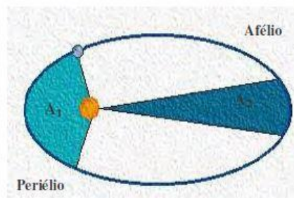
FIGURA 4.19: Para um mesmo intervalo de tempo, os valores das áreas A_1 e A_2 , seriam iguais.
