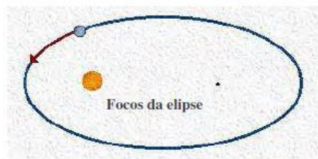
FIGURA 4.18: Representação de uma órbita elíptica.
