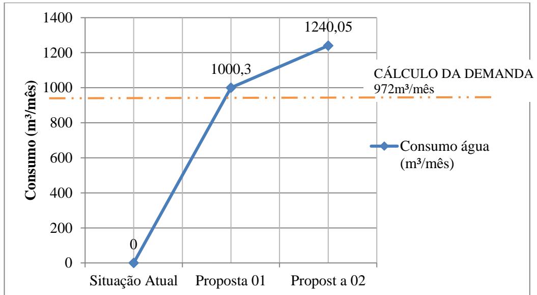
Gráfico 5 - Potencialidade do fornecimento de água de reúso no período de chuvas
