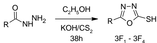
Esquema 23. Síntese de 5-substituído-1,3,4-oxadiazol-2-tiol.
