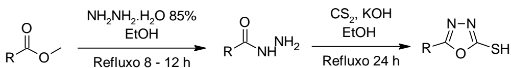
Esquema 27. Síntese do derivado do 1,3,4-oxadiazol.
