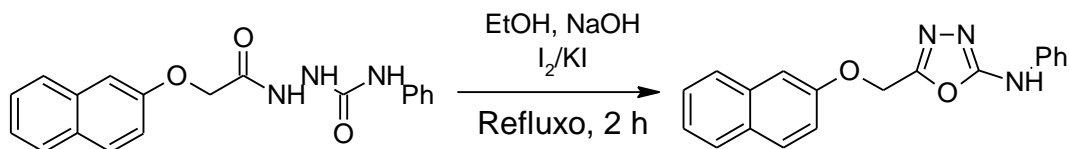
Esquema 15. Obtenção de 1,3,4-oxadiazóis utilizando o iodo como agente desidratante.
