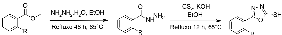
Esquema 24. Síntese do tiol-1,3,4-oxadiazol.
