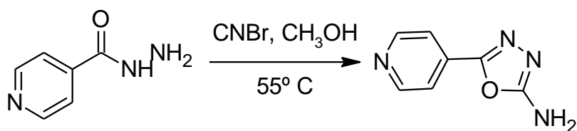
Esquema 11. Síntese de 1,3,4-oxadiazol derivado de isoniazida.
