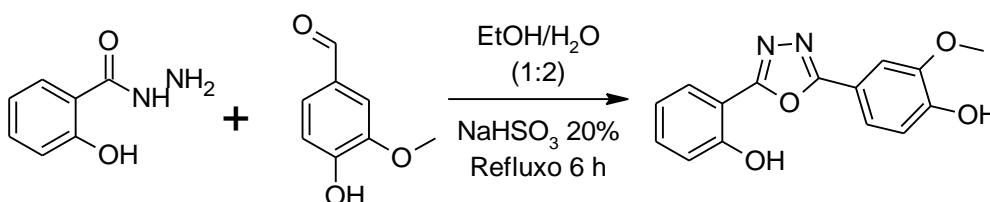
Esquema 40. Tentativa de síntese do 4-[5-(2-hidroxifenil)-1,3,4-oxadiazol-2-il]-2-metoxifenol.
