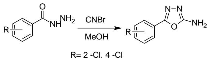
Esquema 12. Síntese de 5-aryl-1,3,4-oxadiazol-2-amino utilizando o brometo de cianogênio.
