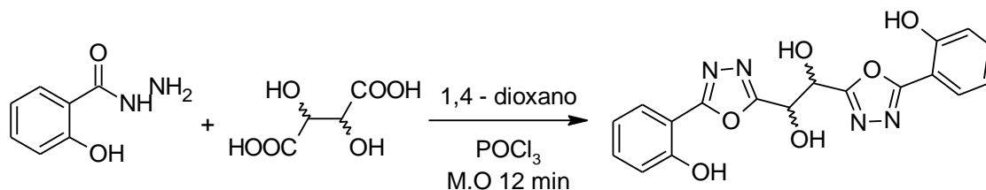
Esquema 35. Tentativa de síntese do 1,2-bis-[5-(2-hidroxifenil)-1,3,4-oxadiazol-2-il] etano-1,2-diol.
