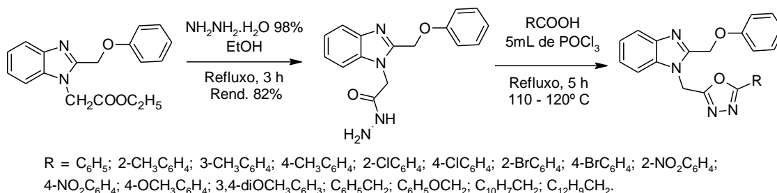
Esquema 16. Síntese 1,3,4-oxadiazóis, utilizando POCl 3 .
