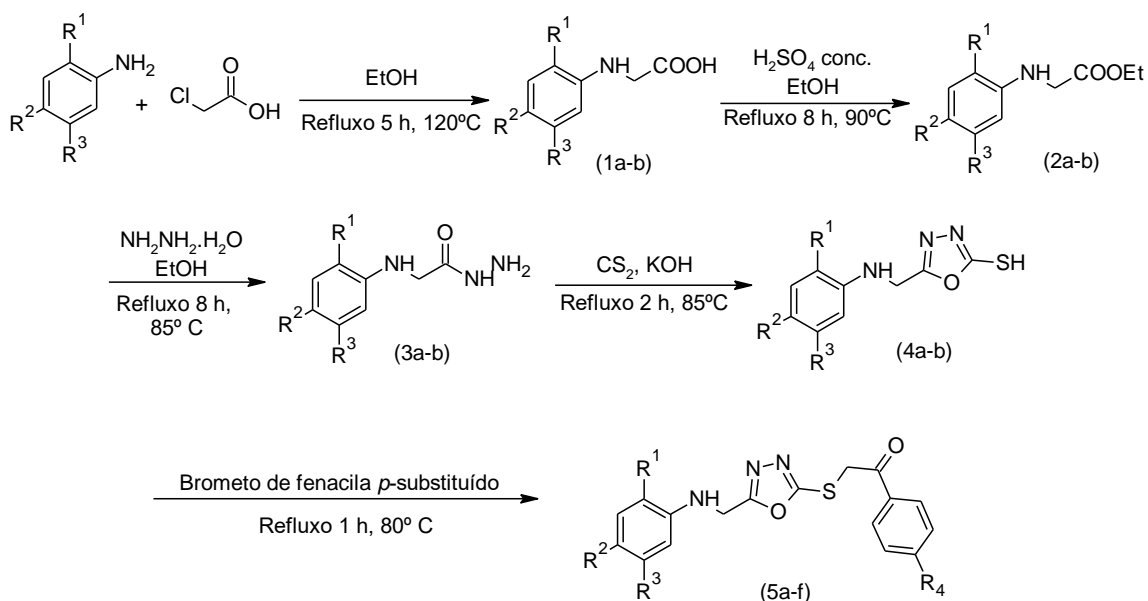
Esquema 25. Síntese dos compostos fenacil-1,3,4-oxadiazol-tiol S-substituídos.
