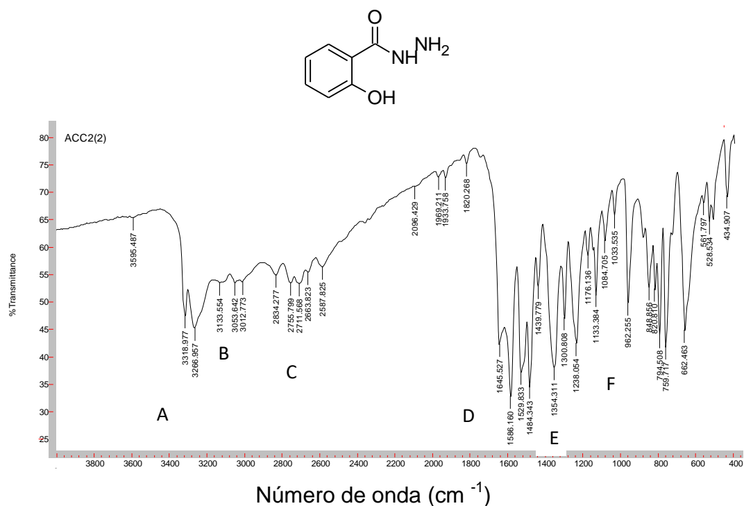
Figura 8. Espectro na região do Infravermelho da 2-hidroxibenzohidrazida (KBr).
