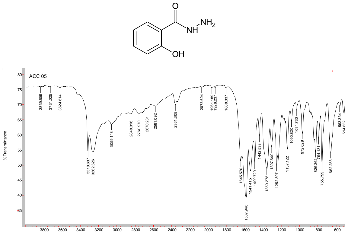
Figura 20. Espectro de FTIR da 2-hidroxibenzo-hidrazida, (KBr).
