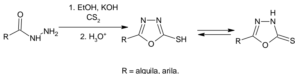
Esquema 22. Síntese de compostos 5-substituído-1,3,4-oxadiazol-2-tiol.
