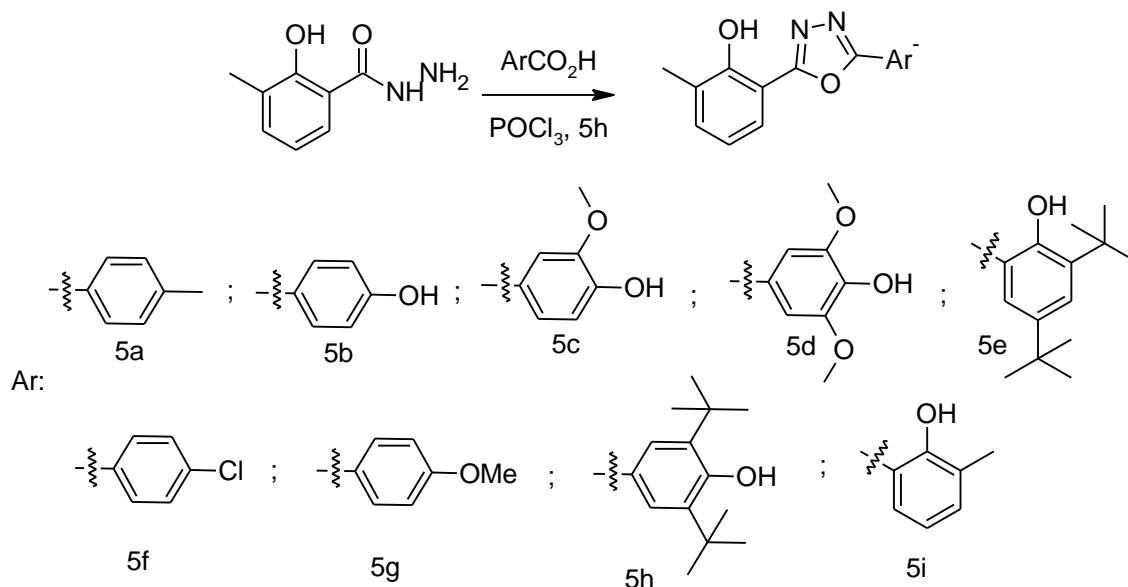
Esquema 21. Síntese de derivados de 1,3,4-oxadiazol com potencial antioxidante e antibacteriano.
