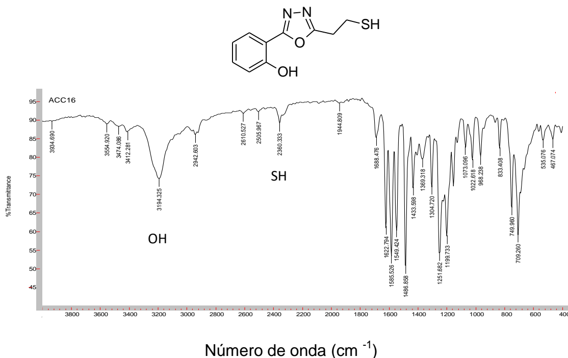
Figura 11. Espectro na região do Infravermelho do 1,3,4-oxadiazol (KBr).
