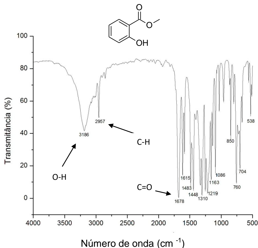
Figura 7. Espectro na região do Infravermelho do salicilato de metila em pastilha de KBr.
