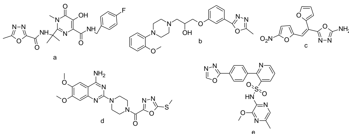
Figura 4. Fórmulas estruturais de Raltegravir(a), Nesapidil(b), Furamisole(c), Tiodazosin(d) e Zibotentan(e).
