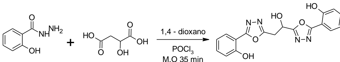
Esquema 36. Tentativa de síntese do 2,2'-[(1-hidroxietano-1,2-diil)-di-1,3,4-oxadiazol-5,2-di-il] difenol.
