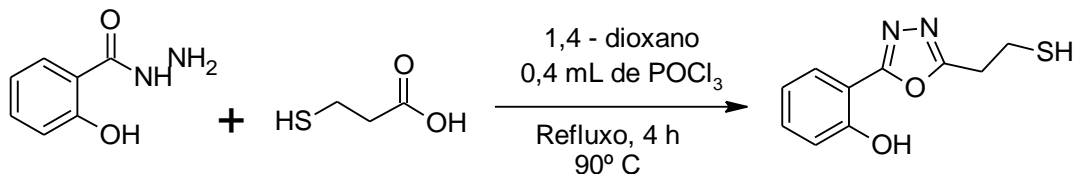
Esquema 31. Síntese do oxadiazol a partir da 2-hidroxi-benzo-hidrazida.
