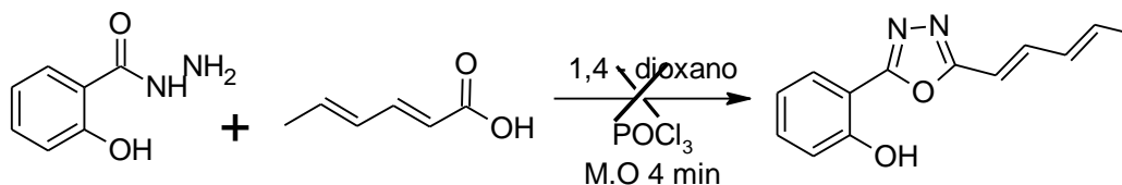
Esquema 39. Tentativa de síntese do 2-[5-[(1 E ,3 E )-penta-1,3-dien-1-il]-1,3,4-oxadiazol-2-il] fenol.
