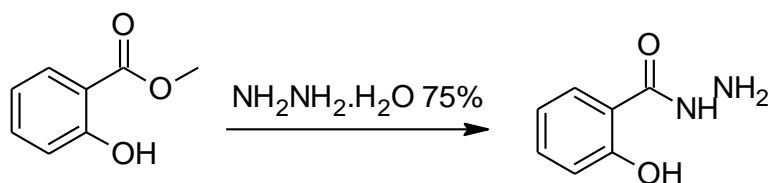
Esquema 3. Obtenção de hidrazida por SMUI.
