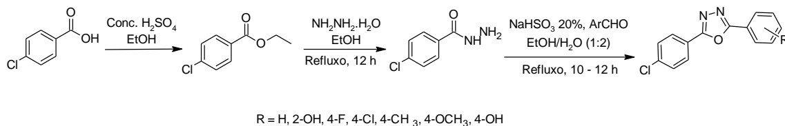
Esquema 17. Síntese de derivados de 1,3,4-oxadiazóis, utilizado NaHSO 3 .
