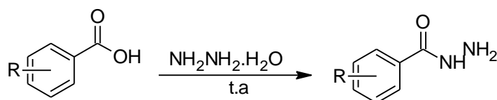
Esquema 4. Síntese de hidrazidas pela técnica de Moagem (marceração).
