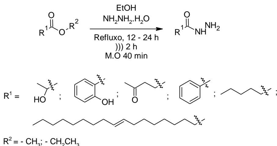
Esquema 29. Síntese das hidrazidas.
