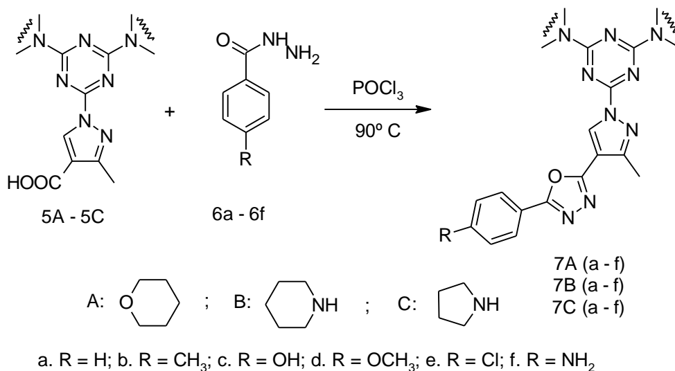
Esquema 20. Síntese de 2,5-dissubstituído-1,3,4-oxadiazol.
