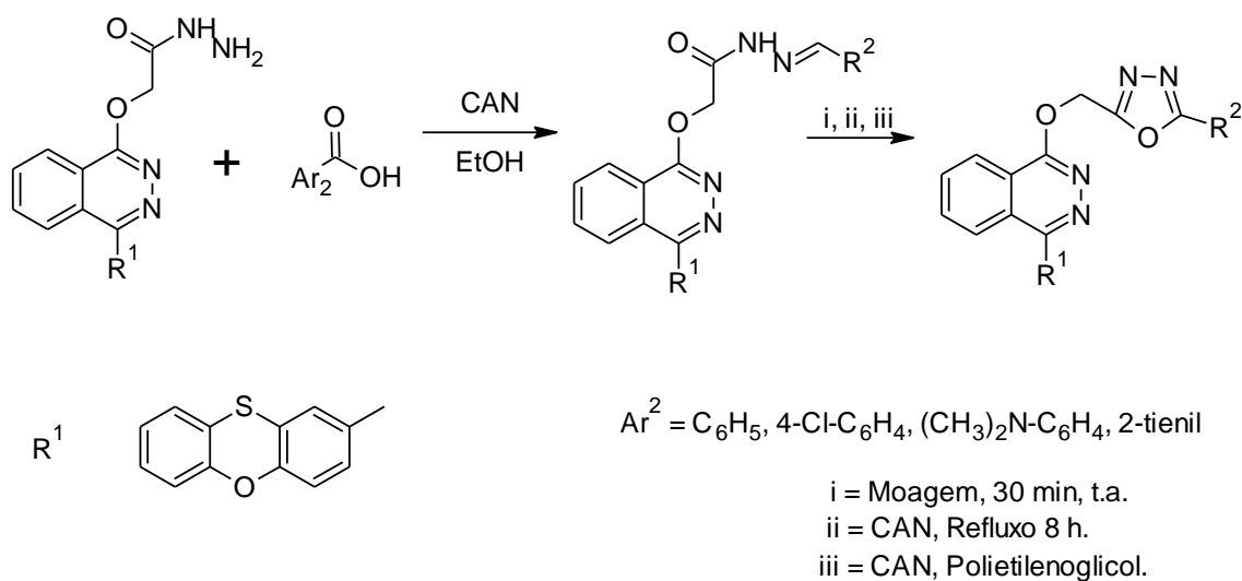
Esquema 19. Síntese de 1,3,4-oxadiazol usando hidrazonas.
