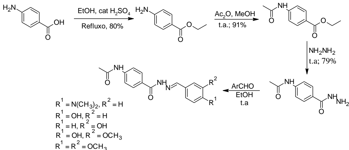
Esquema 10. N -[4-(hidrazinocarbonil)fenil]acetamida como intermediário para obtenção de hidrazonas.
