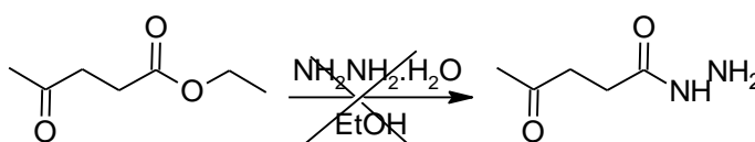
Esquema 33. Síntese da 4-oxopentanohidrazida.
