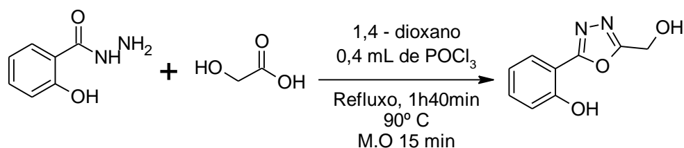
Esquema 32. Síntese do oxadiazol a partir da 2-hidroxibenzo-hidrazida.
