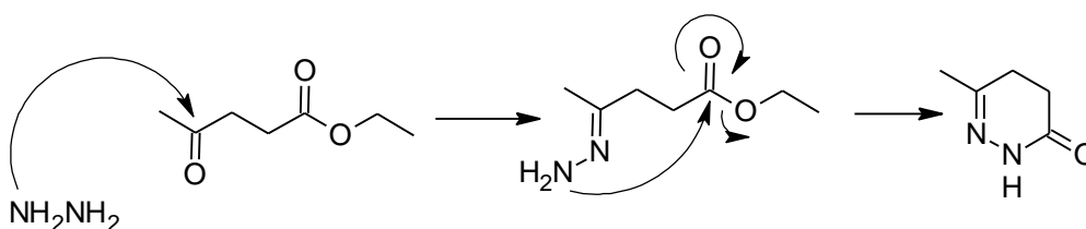
Esquema 34. Proposta sintética da 6-metil-4,5-di-hidropiridazin-3 (2H) –ona.
