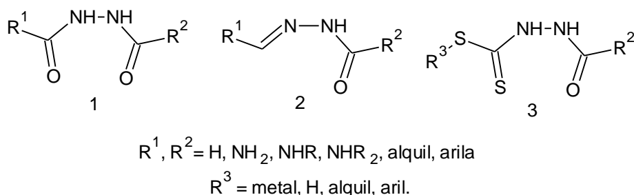
Figura 6. Fórmulas estruturais de diacilhidrazidas (1), acilhidrazonas (2) e ditioatos (3).
