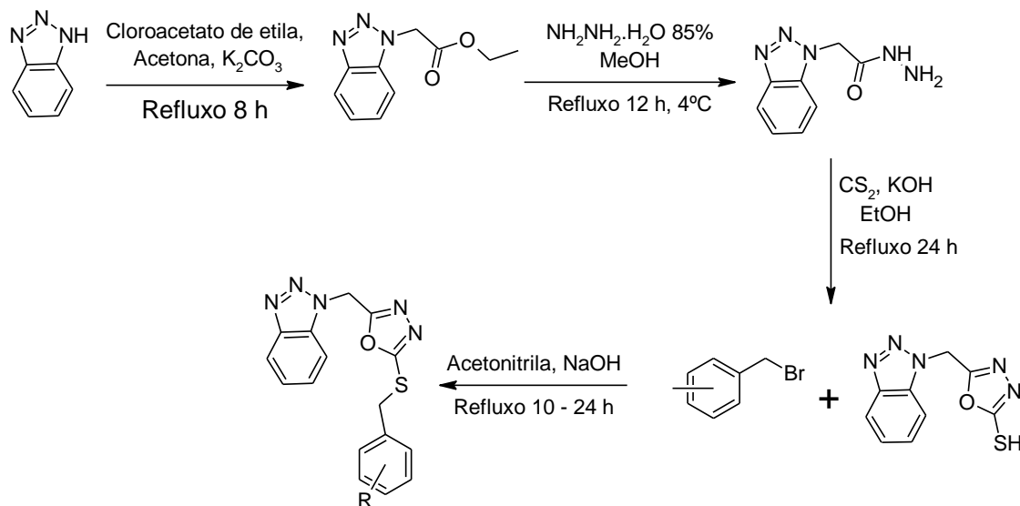
Esquema 26. Derivados de 1,3,4-oxadiazóis contendo o benzotriazol.
