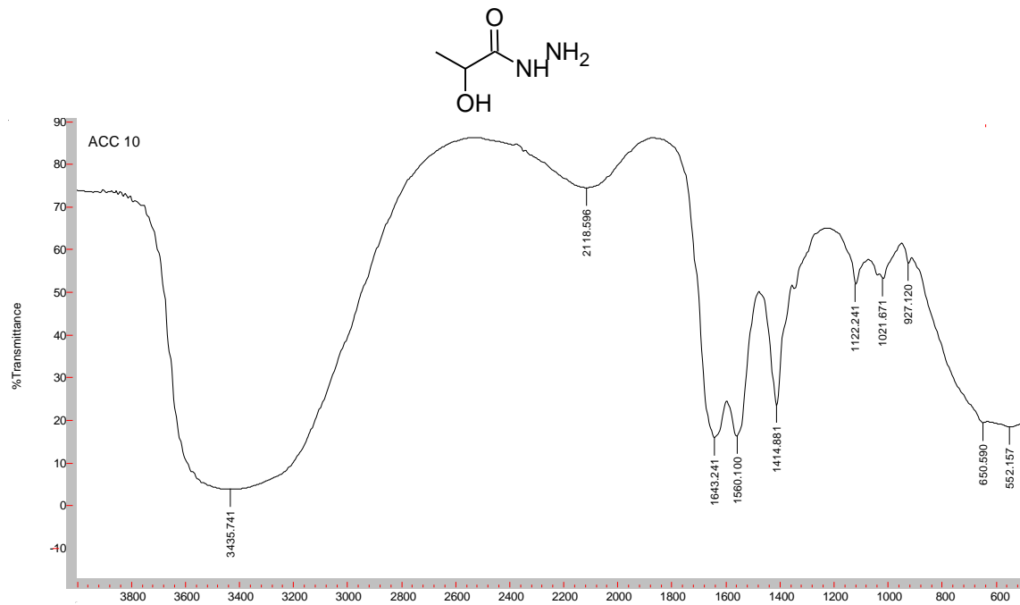
Figura 17. Espectro de FTIR da (2S) -2-hidroxiopropano-hidrazida, (KBr).
