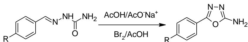
Esquema 14. Síntese de derivados de 1,3,4-oxadiazol por ciclização oxidativa.
