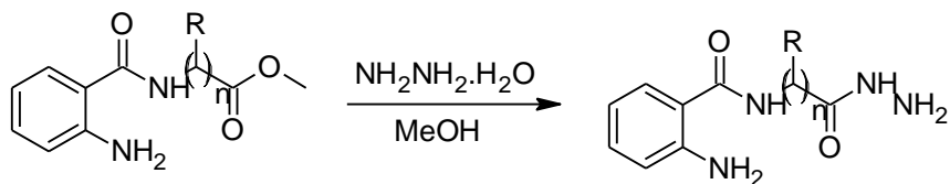
Esquema 5. Síntese de hidrazida em temperatura ambiente.
