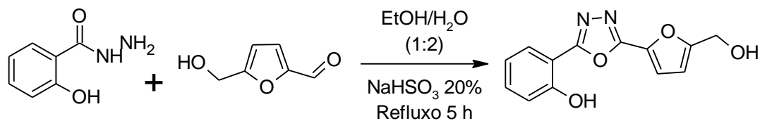
Esquema 41. Tentativa de síntese do 2-[5-[5-(hidroximetil) furano-2-il] -1,3,4-oxadiazol-2-il] fenol.
