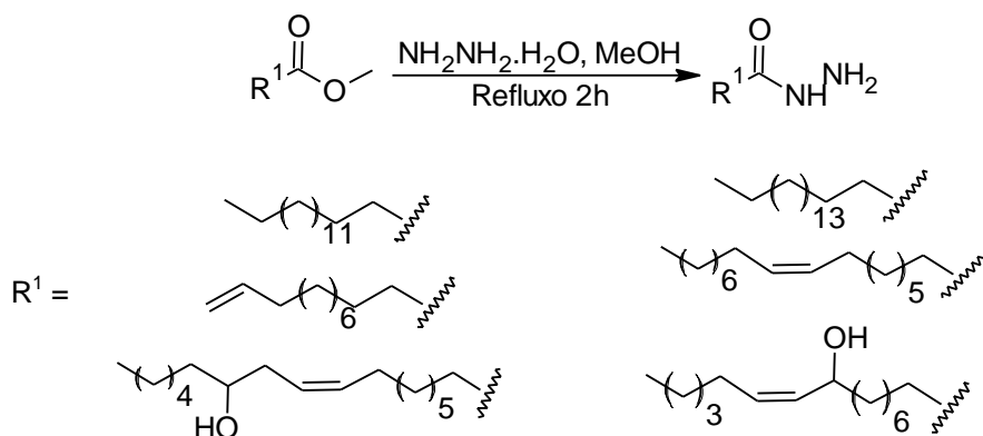
Esquema 6. Hidrazonólise a partir de ésteres graxos.
