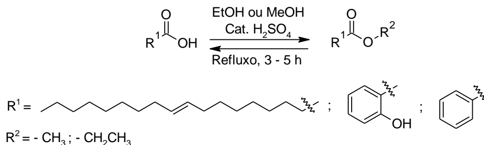
Esquema 28. Reação de esterificação do ácido oleico, salicílico e benzoico.
