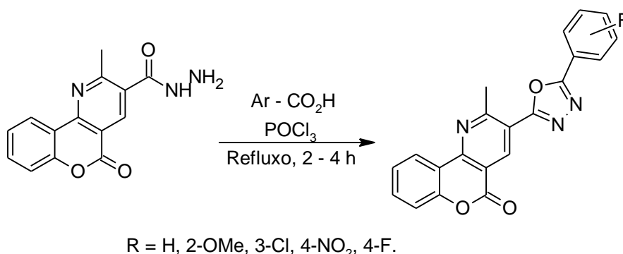
Esquema 18. Síntese de derivados de 1,3,4-oxadiazóis.
