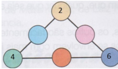
Figura 13 – triângulo com vértices composto de números pares.
