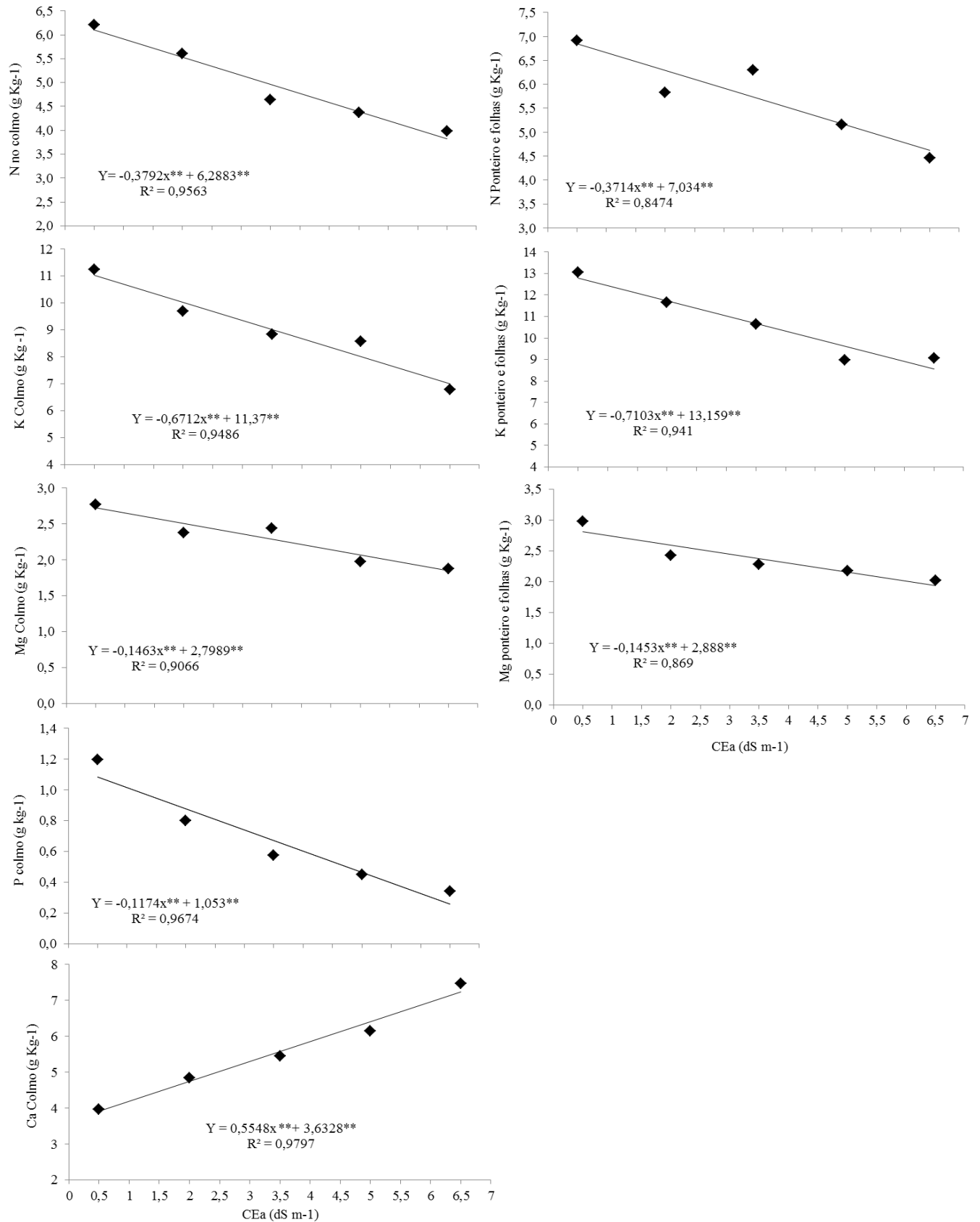
Figura 16. Teores de macronutrientes: nitrogênio (N), fósforo (P), potássio (K), cálcio (Ca) e magnésio (Mg) no colmo e N, K e Mg no ponteiro e folhas da cana-de-açúcar submetidas a diferentes níveis de salinidade da água de irrigação
