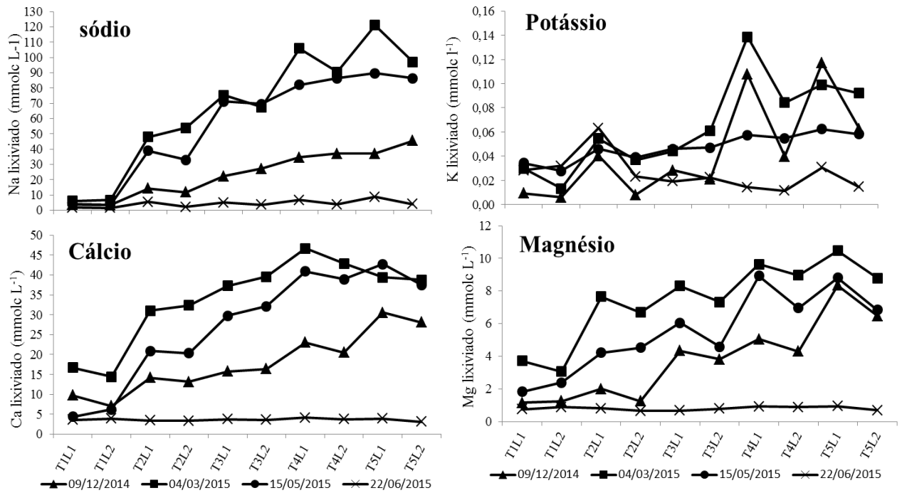
Figura 7. Concentração de sódio; potássio; cálcio e magnésio na água drenada
