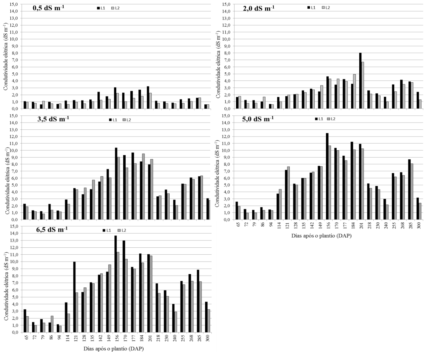
Figura 6. Condutividade elétrica da água drenada nos lisímetros
