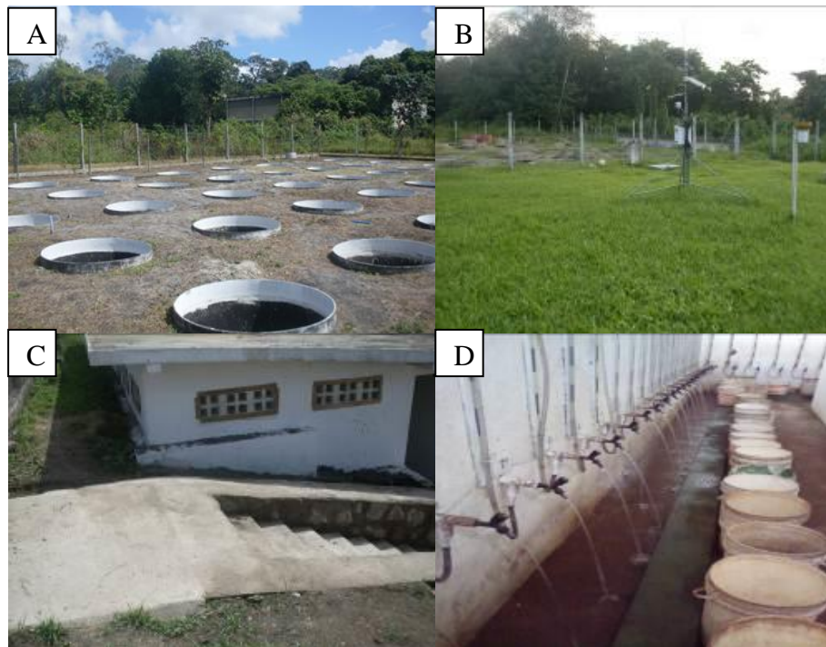
Figura 2. Vista geral dos lisímetros (A); estação meteorológica automática (B); casa de coleta do material drenado (C, D)
