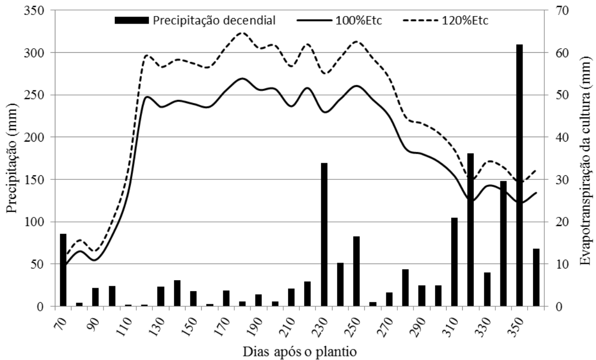
Figura 5. Precipitação e ETC observada durante o experimento
