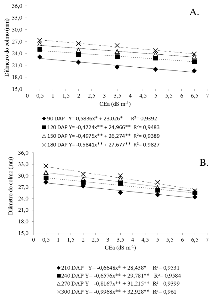
Figura 10. Diâmetro do colmo da cana-de-açúcar submetidas a diferentes níveis de salinidade da água de irrigação em diferentes épocas do ciclo
