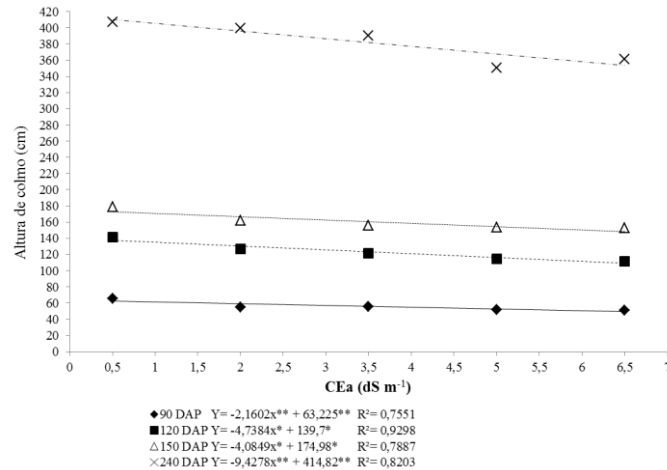
Figura 9. Altura de colmo da cana-de-açúcar submetidas a diferentes níveis de salinidade da água de irrigação em diferentes épocas do ciclo
