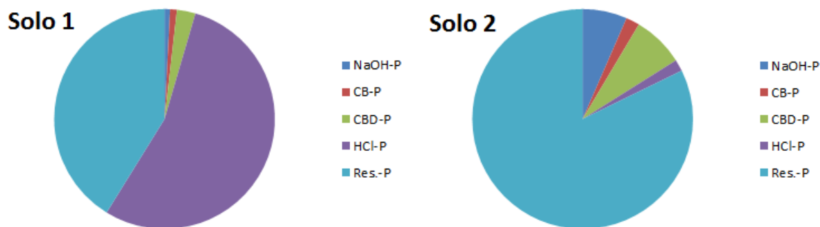
Figura 7 - Porcentagem das frações de P nos cambissolos solódicos (solos 1 e 2)
