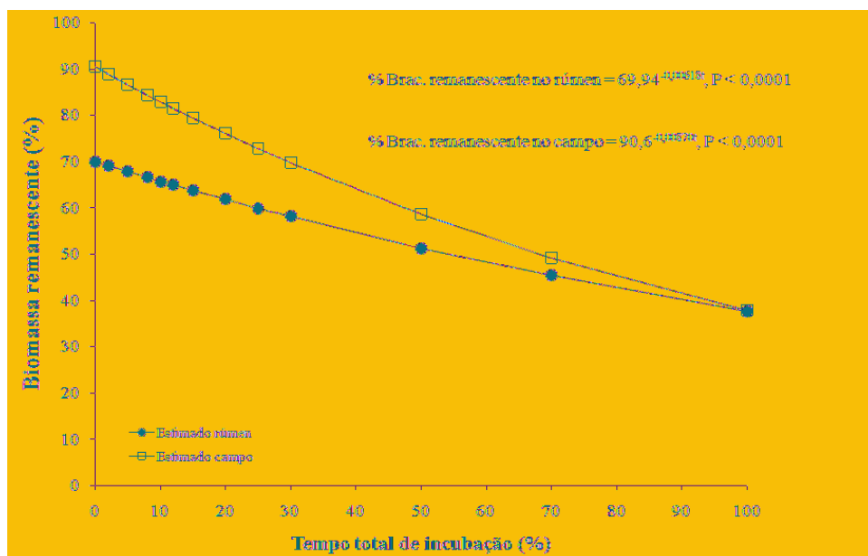
Figura 8. Comparativo da porcentagem de biomassa remanescente no rúmen e no campo na base da matéria seca (MS) de Brachiaria decumbens em escalas de tempos correlacionados, 100% no rúmen = 144 horas; 100% no campo = 256 dias. IC(B0)_{\text{rúmen}}=69,9075-69,9925 ; IC(B0)_{\text{campo}}=90,6-90,6 ; IC(k)_{\text{rúmen}}=0,00615-0,00620 ; IC(k)_{\text{campo}}=0,00870-0,00870 .
