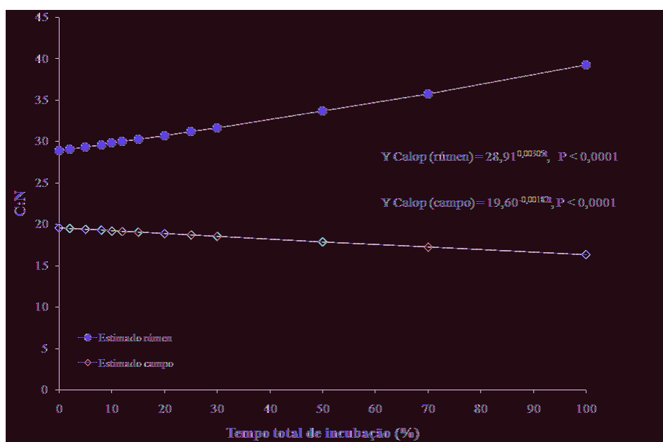
Figura 11. Comparativo da relação C:N no rúmen e no campo na base da matéria seca (MS) de Calopogonium mucunoides em escalas de tempos correlacionados, 100% no rúmen = 144 horas; 100% no campo = 256 dias.
