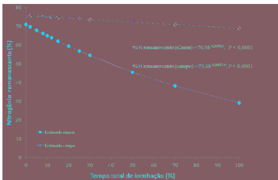
Figura 12. Comparativo da porcentagem de nitrogênio remanescente no rúmen e no campo na base da matéria seca (MS) de Brachiaria decumbens em escalas de tempos correlacionados, 100% no rúmen = 144 horas; 100% no campo = 256 dias. IC(B0)_{\text{rúmen}}=70,9262-71,0370 ; IC(B0)_{\text{campo}}=75,6800-75,6800 ; IC(k)_{\text{rúmen}}=0,00883-0,00889 ; IC(k)_{\text{campo}}=0,000924-0,000924 .
