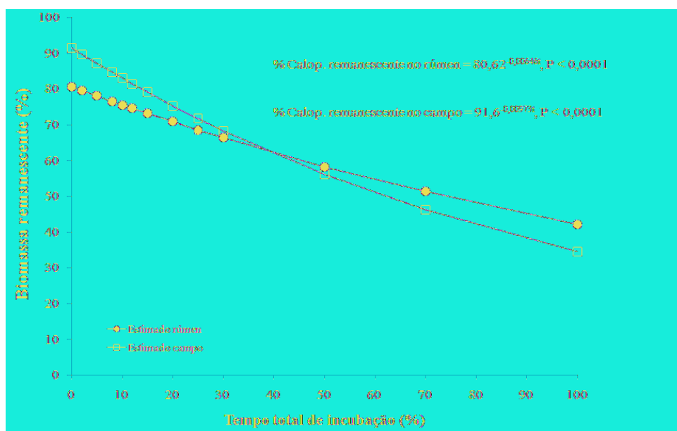
Figura 9. Comparativo da porcentagem de biomassa remanescente no rúmen e no campo na base da matéria seca (MS) de Calopogonium mucunoides em escalas de tempos correlacionados, 100% no rúmen = 144 horas; 100% no campo = 256 dias. IC(B0)_{\text{rúmen}}=80,5711-0,6724 ; IC(B0)_{\text{campo}}=91,6-91,6 ; IC(k)_{\text{rúmen}}=0,00644-0,00648 ; IC(k)_{\text{campo}}=0,00973-0,00973 .
