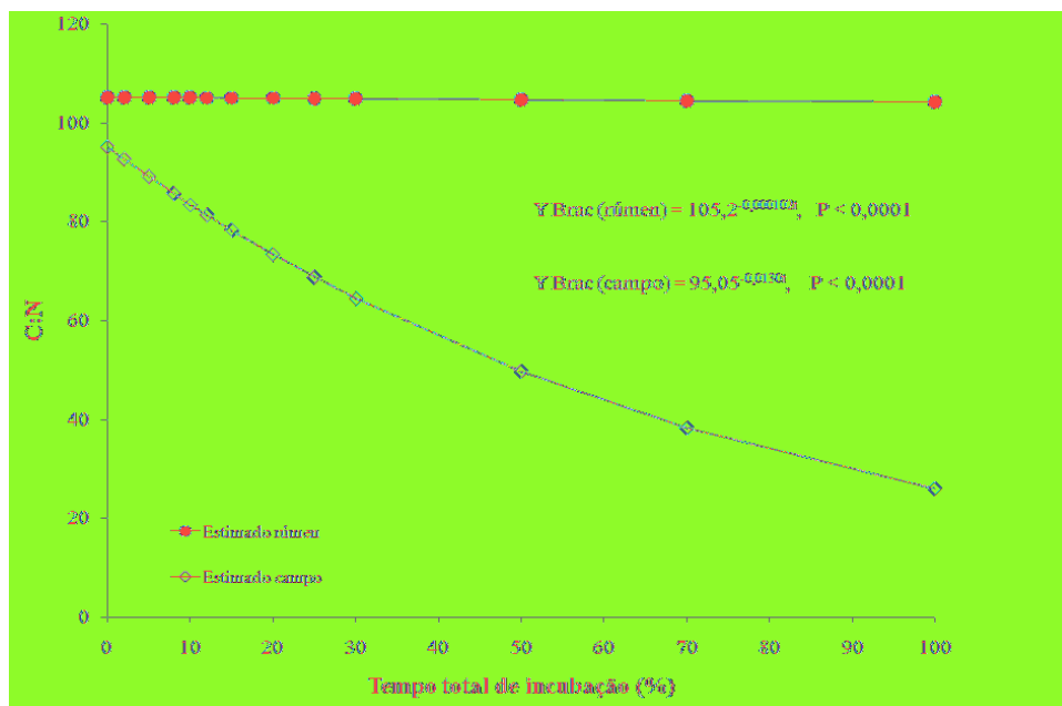
Figura 10. Comparativo da relação C:N no rúmen e no campo na base da matéria seca (MS) de Brachiaria decumbens em escalas de tempos correlacionados, 100% no rúmen = 144 horas; 100% no campo = 256 dias. IC(B0)_{rúmen}=105,2-105,2 ; IC(B0)_{campo}=95,05-95,05 ; IC(k)_{rúmen}=0,000102-0,000102 ; IC(k)_{campo}=0,0130-0,130 .
