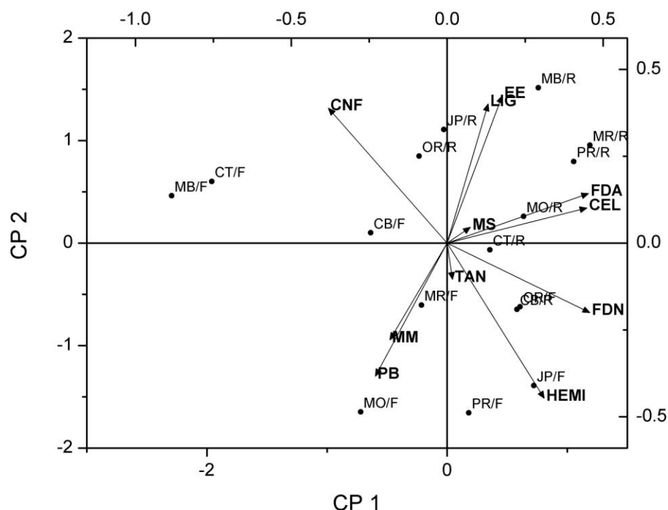
Figura 5. Biplot dos primeiros componentes principais dos vetores de cargas (variáveis) e dos escores (espécie/componente morfológico) no mês de abril de 2011.
