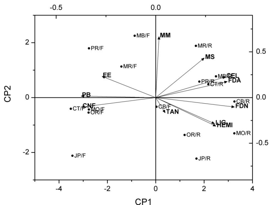
Figura 3. Biplot dos primeiros componentes principais dos vetores de cargas (variáveis) e dos escores (espécie/componente morfológico) no mês de janeiro de 2011.
