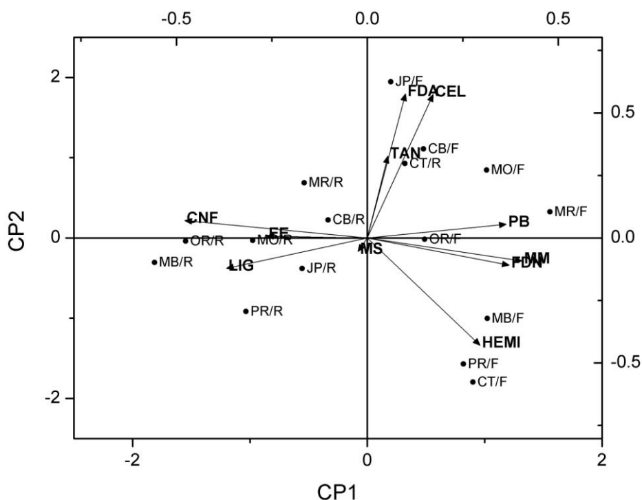
Figura 7. Biplot dos primeiros componentes principais dos vetores de cargas (variáveis) e dos escores (espécie/componente morfológico) no mês de agosto de 2011.
