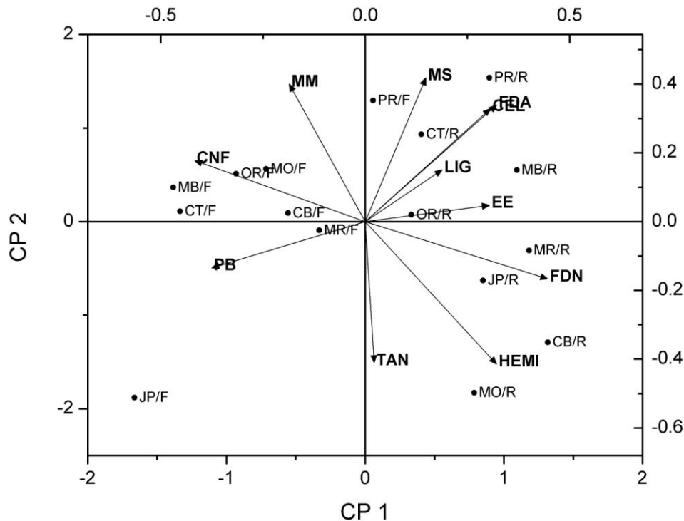
Figura 4. Biplot dos primeiros componentes principais dos vetores de cargas (variáveis) e dos escores (espécie/componente morfológico) no mês de março de 2011. Variáveis: MS=matéria seca, MM=matéria mineral, PB=proteína bruta, CEL=celulose, HEM=hemicelulose, LIG= lignina, EE=extrato etéreo, CNF=carboidratos não fibrosos, TC=taninos condensados, FDN=fibra em detergente neutro e FDA=fibra em detergente ácido. Espécies: MB=malva branca, MR= marmeleiro, CB= capa bode, CT= catingueira, PR= pereiro, MO=mororó, JP=jurema preta, OR=orelha de onça, sendo F para folha e R para ramo.
