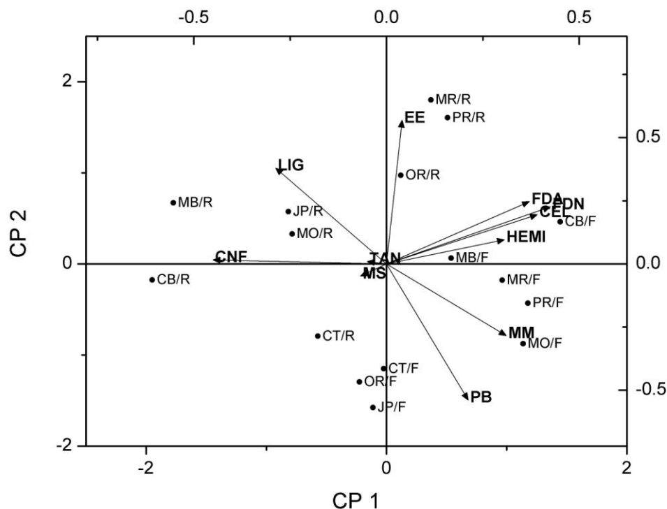
Figura 6. Biplot dos primeiros componentes principais dos vetores de cargas (variáveis) e dos escores (espécie/componente morfológico) no mês de junho de 2011.
