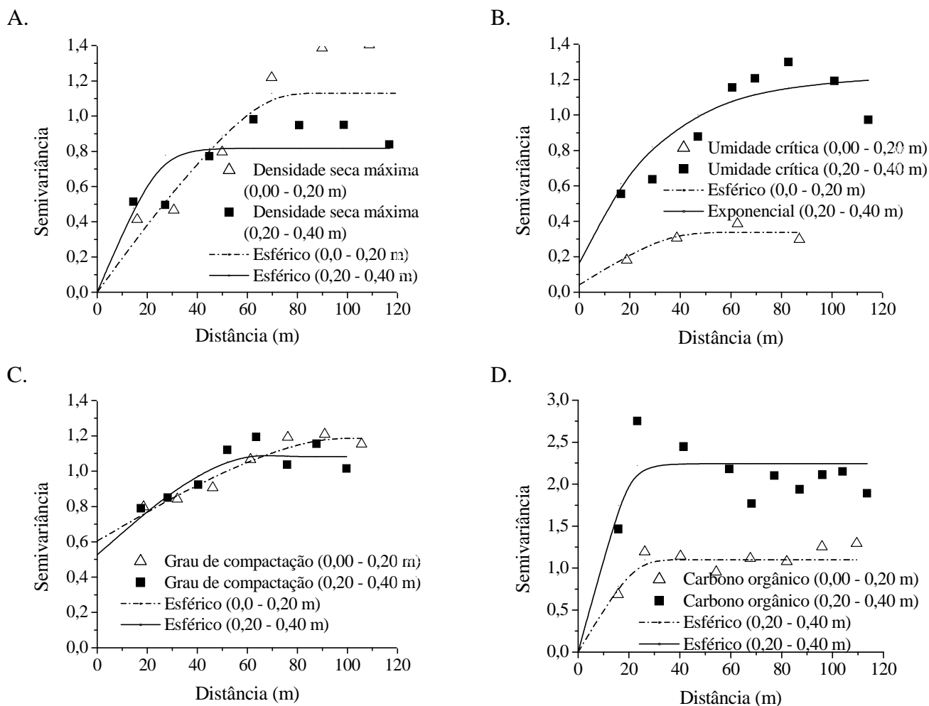
Figura 12. Semivariogramas Densidade seca máxima (A), Umidade crítica (B), grau de compactação (C) e Carbono orgânico (D)
