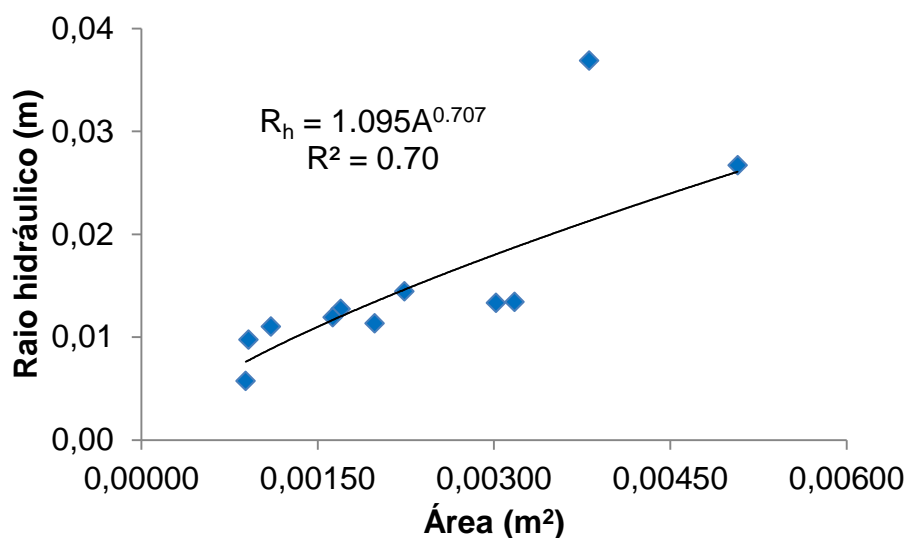
Figura 28. Relação exponencial entre a área e o raio hidráulico dos sulcos gerados pelos fluxos crescentes aplicados na avaliação da erosão em sulcos sobre o Cambissolo estudado.
