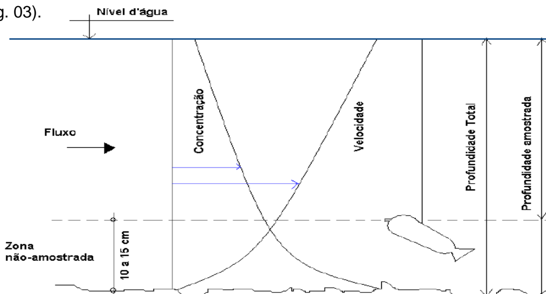
Figura 03 – Zona de amostragem, medida e não medida, numa vertical de amostragem de sedimento em suspensão, Guy e Norman (1970). apud Santos et al. (2001). Modificado.
