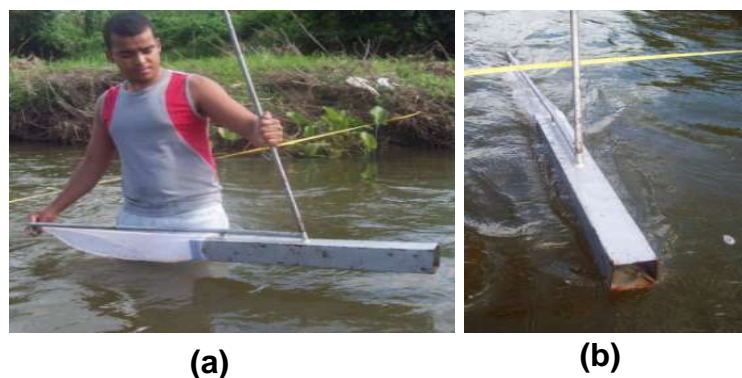
Figura 9 – Coleta a vau com o amostrador US BLH-84 (a) e detalhamento do amostrador (b).
