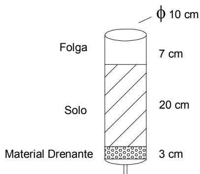
Figura 2. Esquema do vaso de PVC empregado no cultivo das plantas.
