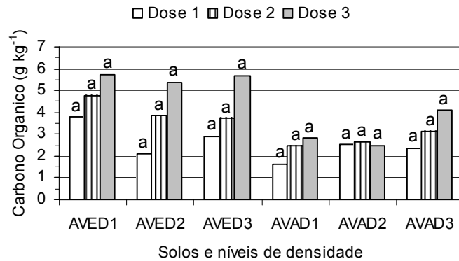
Figura 8. Teores de CO no solo após a aplicação de diversas dosagens do composto orgânico em função do tipo de solo e densidades.
