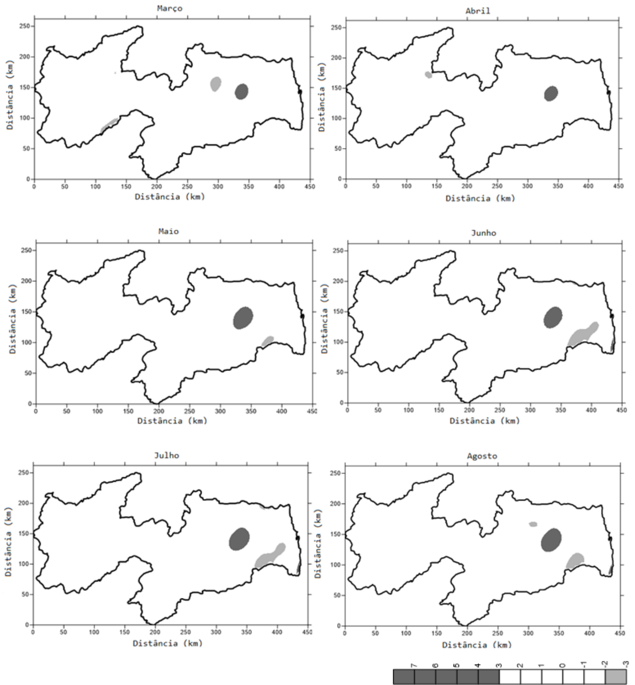
Figura 5.6: Mapas dos resíduos padronizados das diferenças entre os valores observados e estimados pelas superfícies de 3ª e 4ª ordem da precipitação pluvial do Estado da Paraíba.
