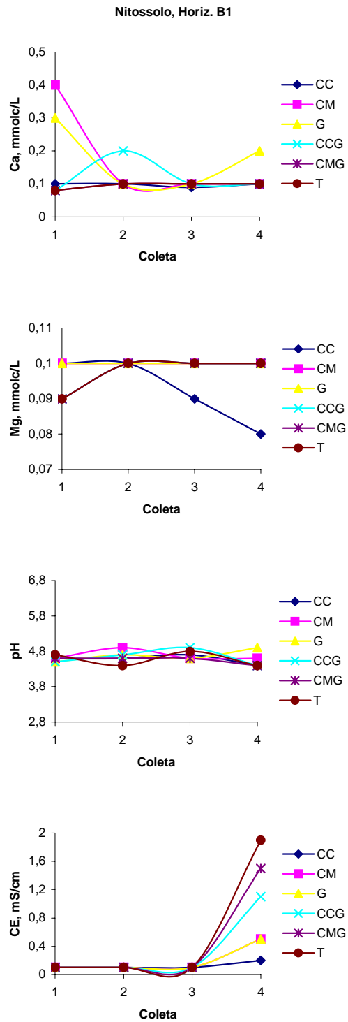
Figura 5. Teores de cálcio, magnésio e valores de pH e condutividade elétrica do lixiviado das amostras do Nitossolo Horizonte B1, nas quatro coletas.
