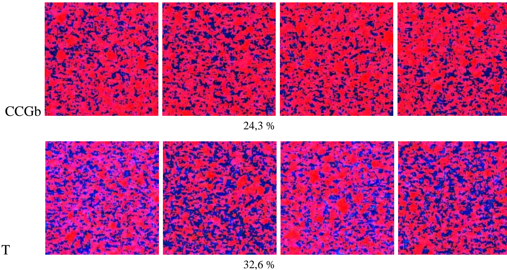
Figura 10 - Imagens com dimensões de 5,64 x 5,74 cm tomadas das partes mais uniformes dos blocos impregnados e iluminados com luz ultravioleta. As partes azuis correspondem à porosidade e as vermelhas a matriz do solo. Devido a baixa resolução das imagens a porosidade mínima detectada foi de apenas 352 \mu m. Os números abaixo de cada imagem correspondem ao percentual de espaço poroso calculado. * t – topo; b – base.
