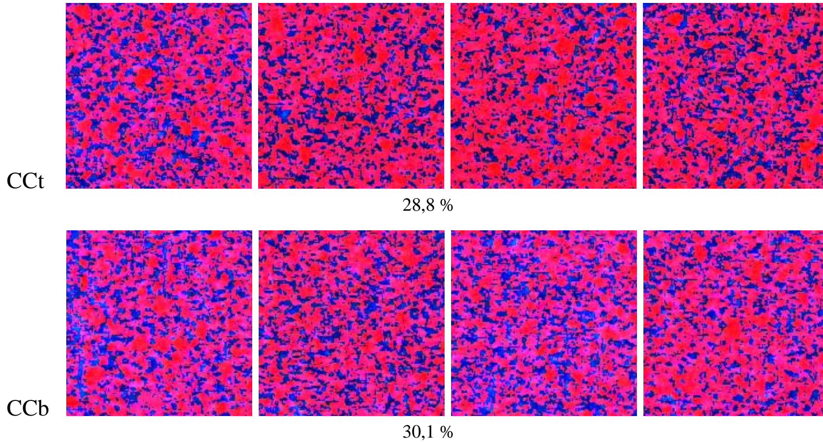
Figura 7 - Imagens com dimensões de 5,64 x 5,74 cm tomadas das partes mais uniformes dos blocos impregnados e iluminados com luz ultravioleta. As partes azuis correspondem à porosidade e as vermelhas a matriz do solo. Devido a baixa resolução das imagens a porosidade mínima detectada foi de apenas 352 \mu m.. Os números abaixo de cada imagem correspondem ao percentual de espaço poroso calculado. * t – topo; b – base.
