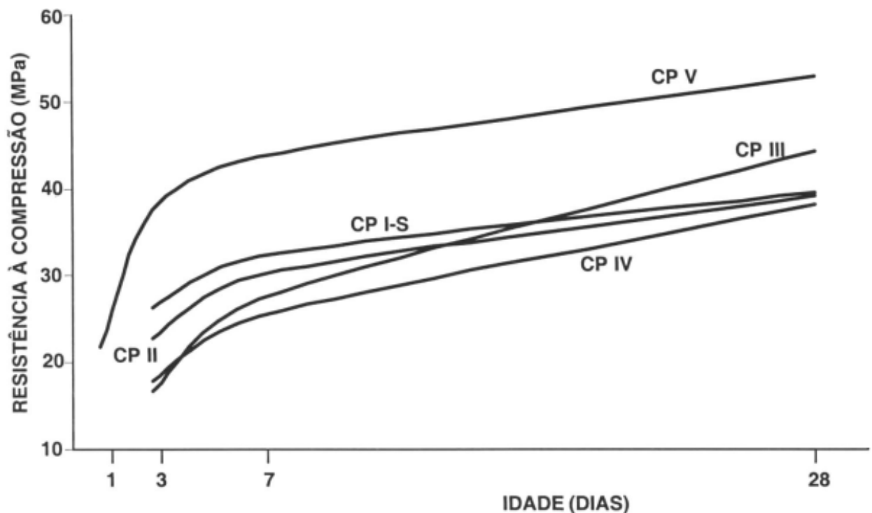
Figura 2. Evolução média de resistência à compressão dos tipos de cimento Portland. Fonte ABCP (2002).
