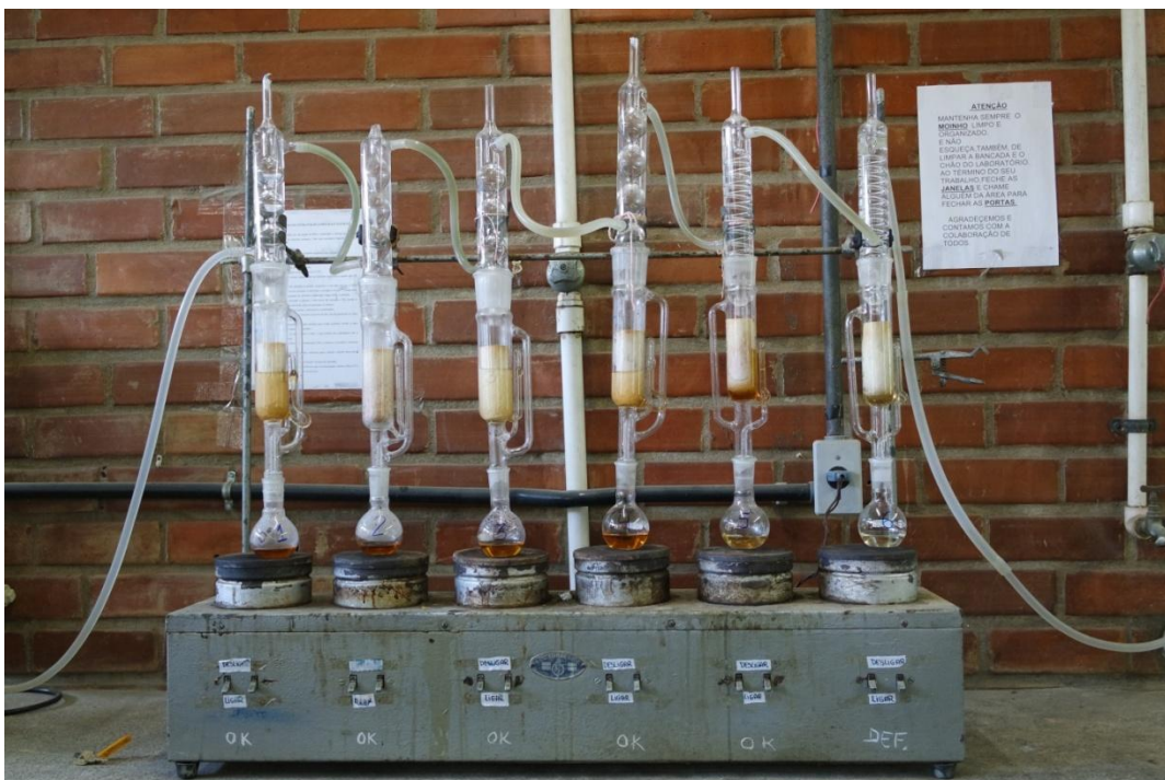
Figura 4. Aparato de extração química Soxhlet.
