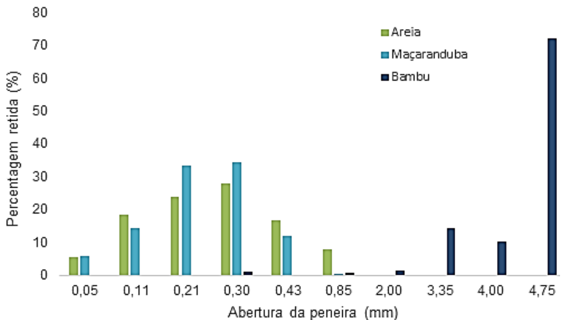
Figura 11. Histograma das percentagens retidas nas peneiras para a areia, Maçaranduba e Bambu.
