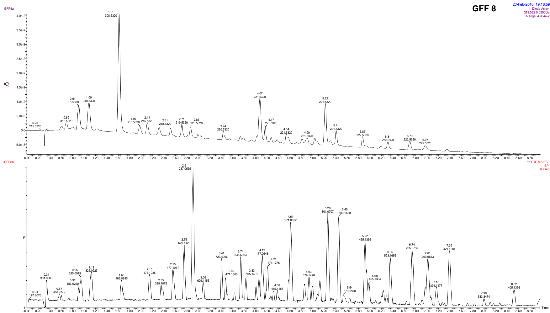
Figura 4. Cromatogramas (UHPLC-PDA, 320 nm) das frações fenólicas de geoprópolis (GFF).
